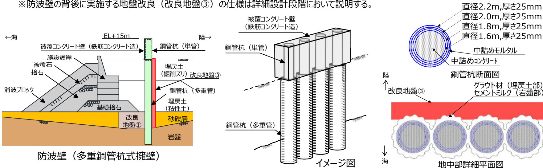
地中部詳細平面図
