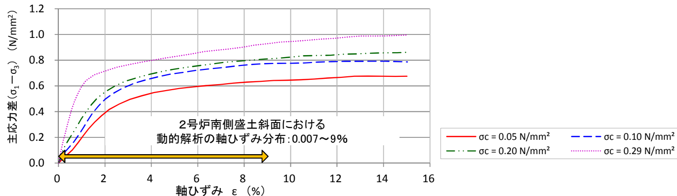
2号炉南側盛土斜面における 動的解析の軸ひずみ分布:0.007~9% 大型三軸圧縮試験結果(応力-ひずみ関係)
