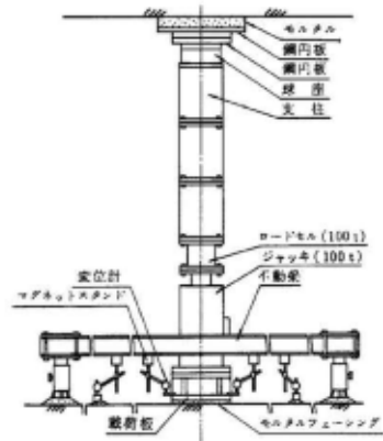
平板載荷試験装置
