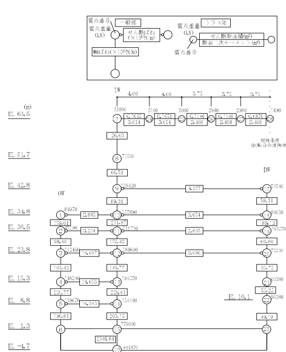
鉛直モデル
