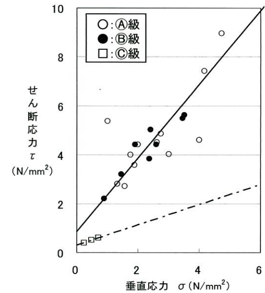
岩盤せん断試験結果(砂岩)
