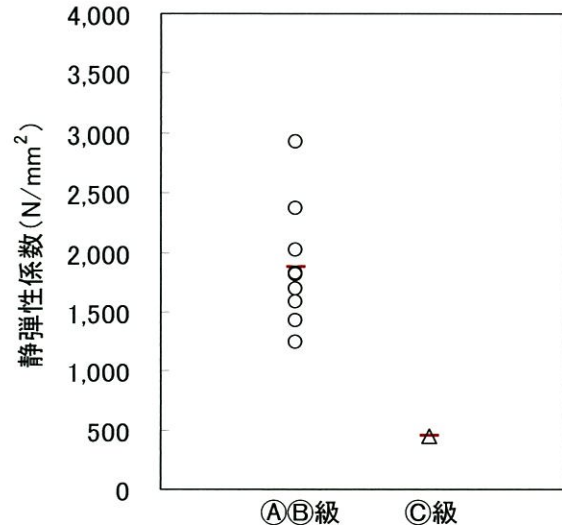
岩盤変形試験結果(砂岩)
