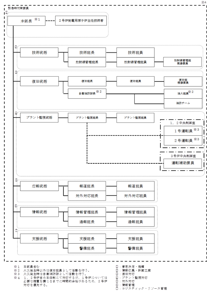
第 2.1 図 原子力防災組織 (島根原子力発電所) (新規制基準として申請している組織を示す)
