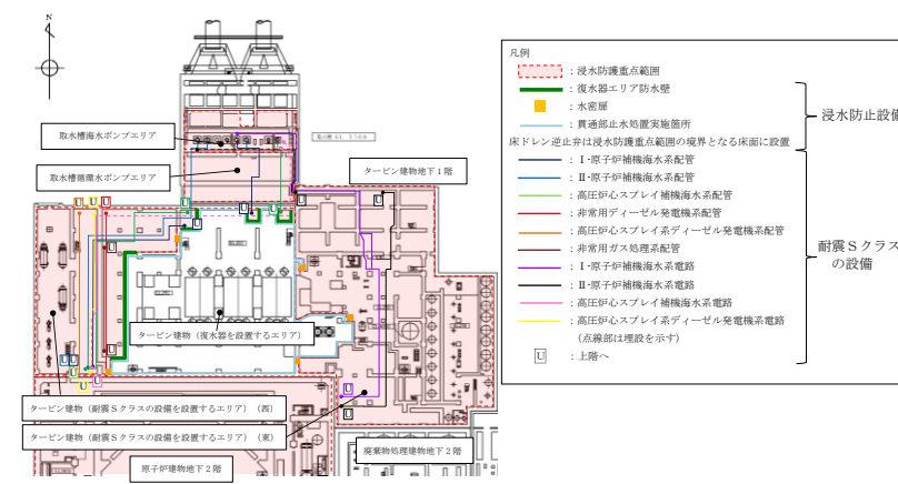
図2 浸水防護重点化範囲内の耐震Sクラスの設備の位置
