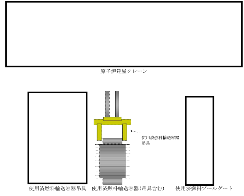
第3.2.5 図 原子炉建屋クレーン本体及び取り扱い設備（6号炉）
