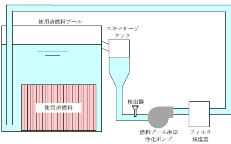
第1.2-7 図 燃料プール冷却浄化系ポンプ入口温度の設置図
