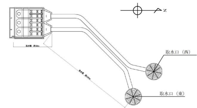
第4-6図 取水口～取水ピット平面図
