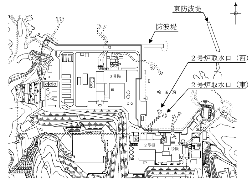
第4-5図 取水口、防波堤及び東防波堤の位置
