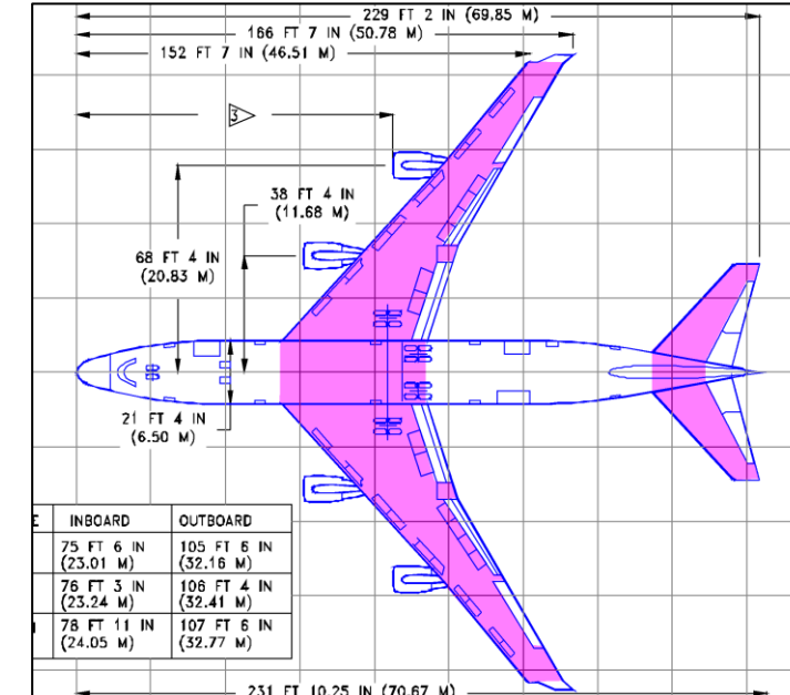
第 1-1(a)図 燃料タンク投影面積 (B747-400)
