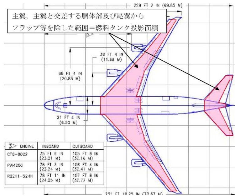
第 1-1(a)図 燃料タンク投影面積(B747-400)
