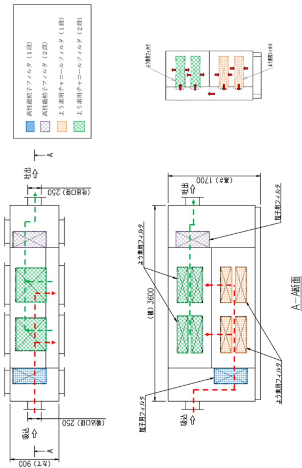
第 2.4-6 図 緊急時対策所空気浄化フィルタユニットの概要図
