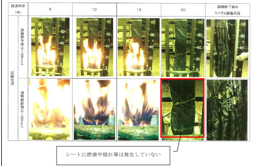
第 2 図 防火シートの IEEE383 垂直トレイ燃焼試験実施後の状態
