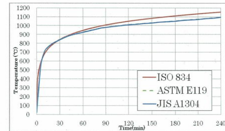
第2図 加熱曲線の比較
