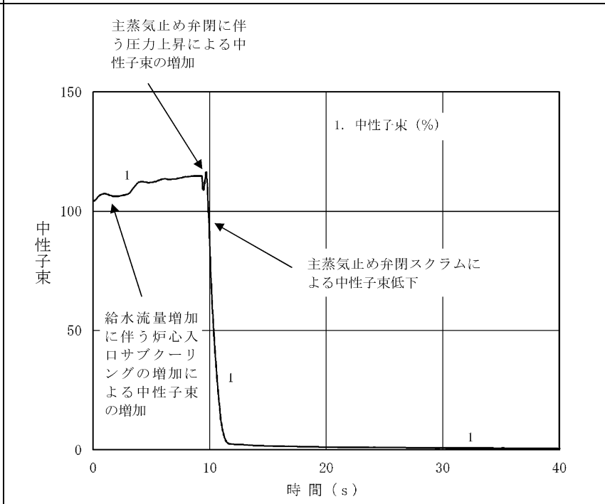
図 6-6 R/Bにおける内部溢水による事象変化 (中性子束) (給水制御系の故障)
