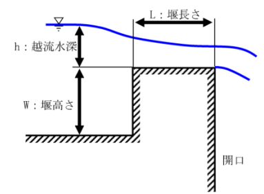
長方堰の越流量 (「水理公式集」より)
