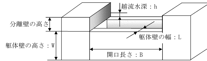
第 10.3-1 図 海水ポンプエリアモデル図
