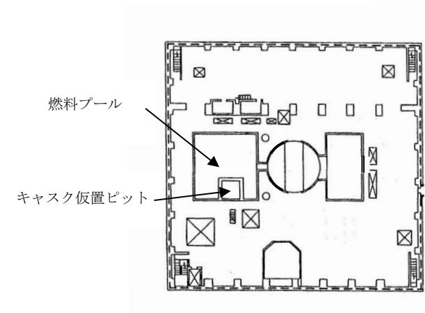
図 8-1 原子炉建物 4 階の機器配置図
