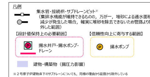
図10-6 地下水低下設備の構成例
