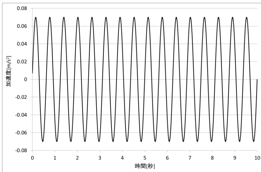
図3-3 入力加振波
