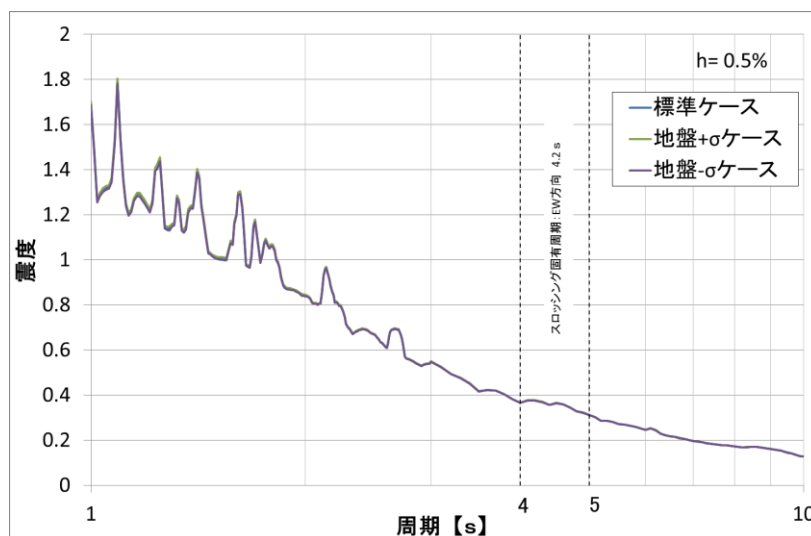
EW 方向
