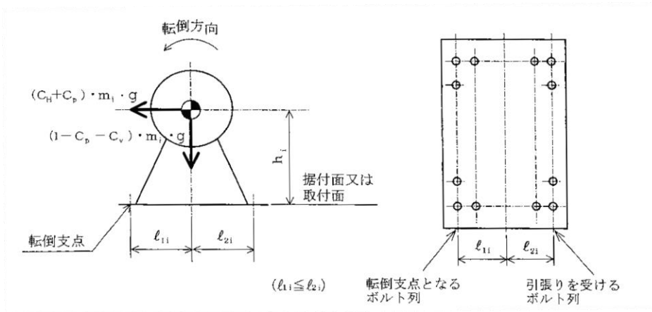
軸直角方向
