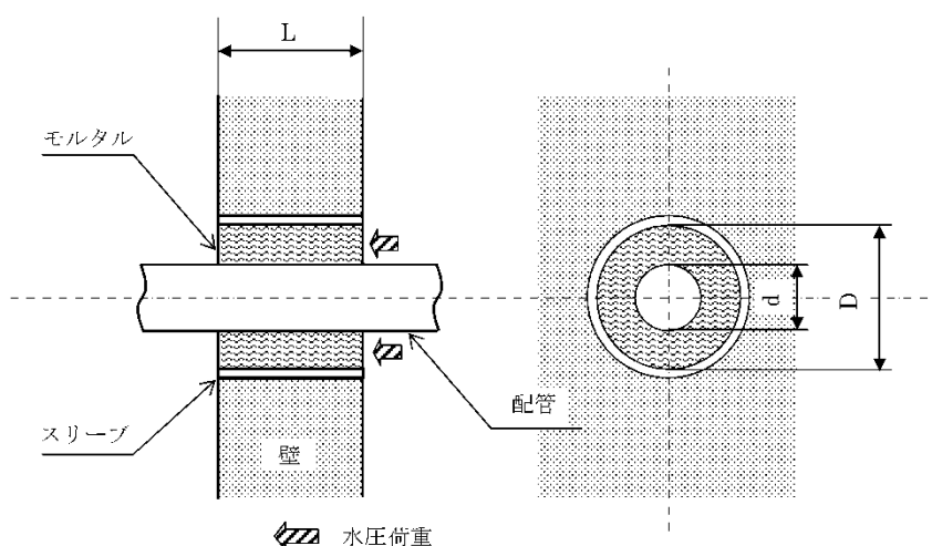
図 2-16 モルタル評価概要図
