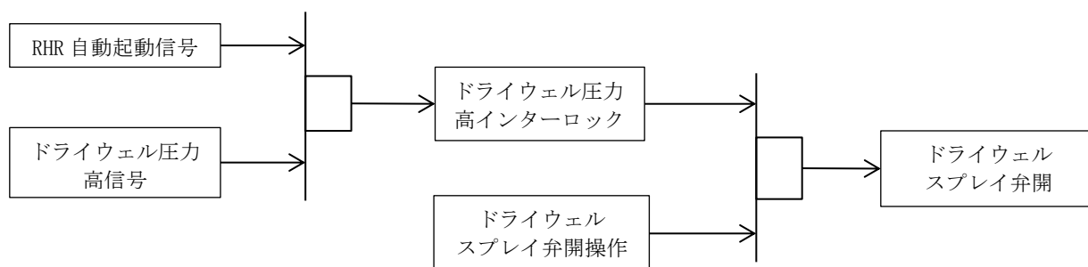
図 3-2 ドライウエルスプレイ弁開インターロック
