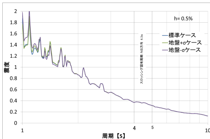
NS 方向
