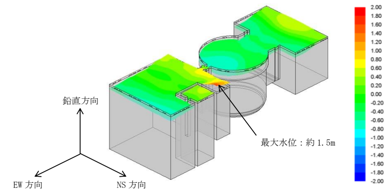
(2) 解析ケース② (EW 方向 + 鉛直方向)
