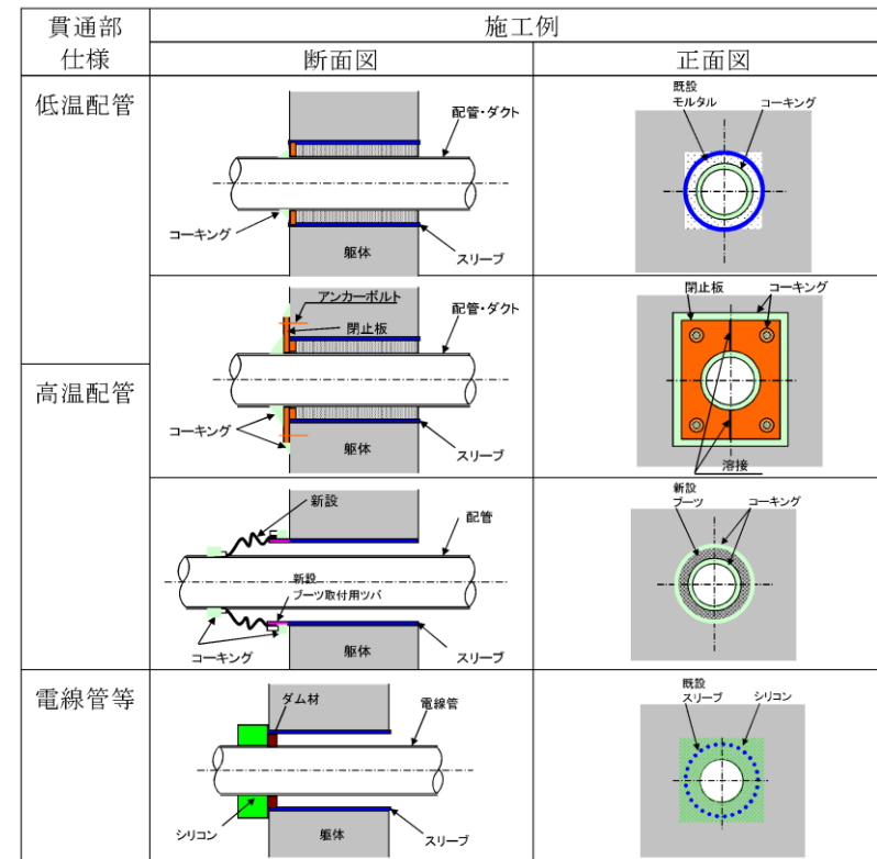
第1図 貫通部止水対策 (施工例)
