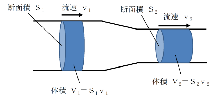
図 2-5 流路断面積と流速の関係
