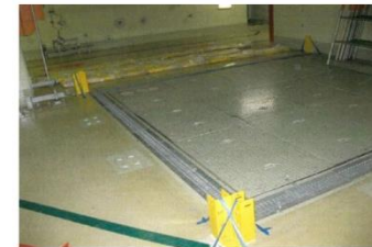
支柱レールの取付状況
