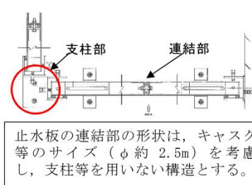
支柱レールの取付状況
