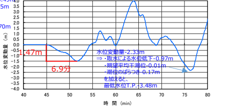
図 1 5 崩壊規模のパラメータスタディ結果 (津波襲来の判断基準 (トリガー) による検知可否の確認)
