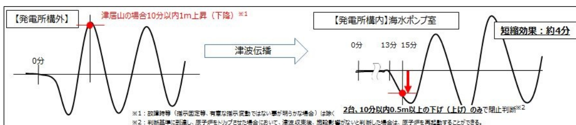
図1 発電所構外にて「プラント影響のある津波」を確認した場合の対応の概念図
