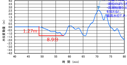
図 1 5 崩壊規模のパラメータスタディ結果 (津波襲来の判断基準 (トリガー) による検知可否の確認)
