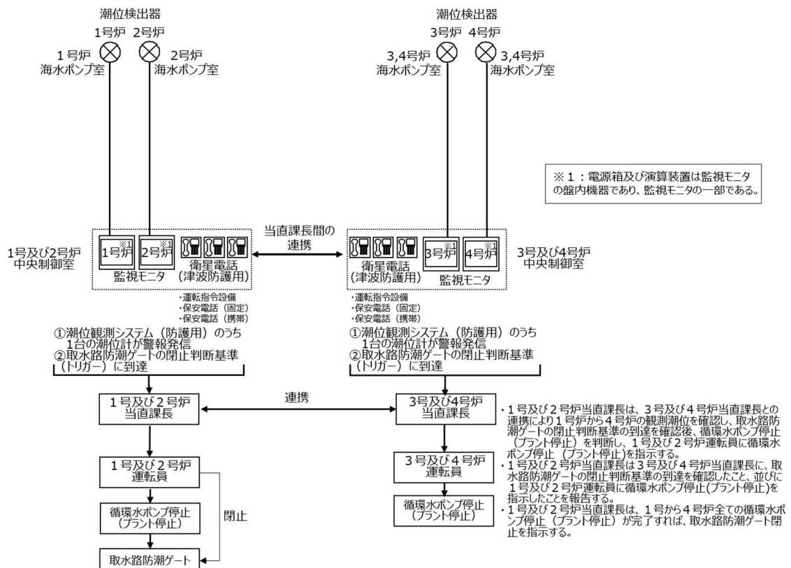
図3 取水路防潮ゲートの閉止判断基準（トリガー）に到達したことを確認するための一連の設備
