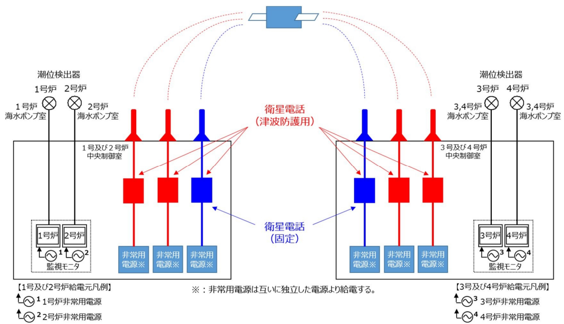
図 2 5 潮位観測システム（防護用）の電源概要図
