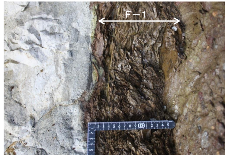
①露頭上方で幅の狭くなる箇所の葉片状破碎部。全体にセピオライト化が進行し、硬質な葉片を主体とする。一部軟質化するが、下方に連続せず風化によるものと判断される。
