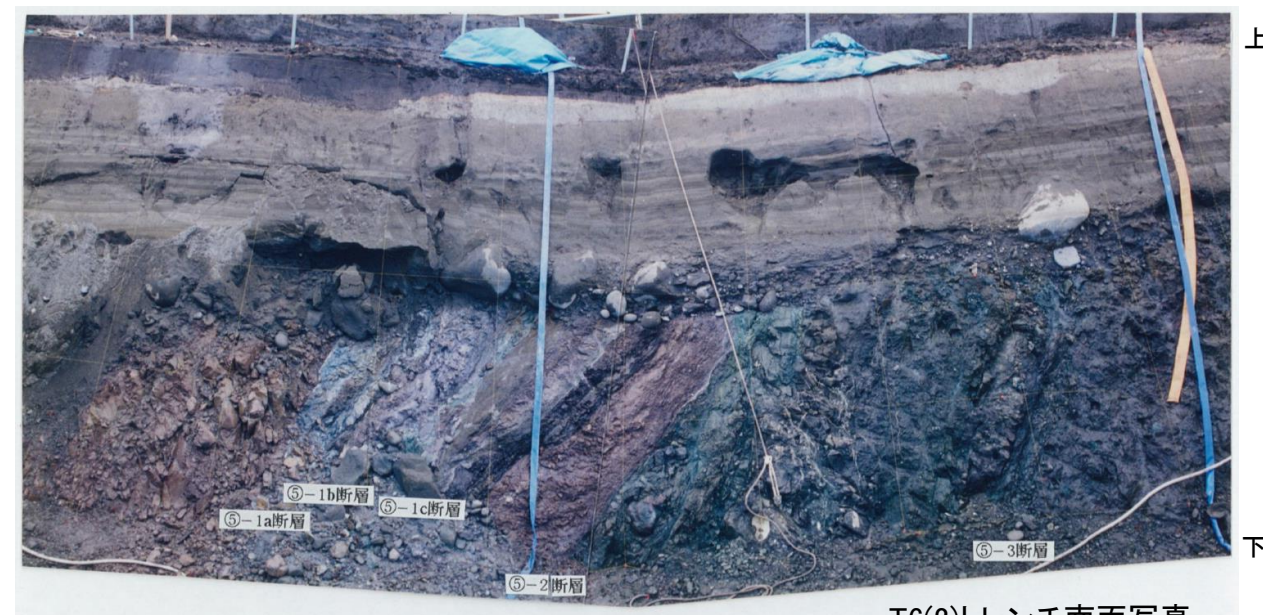
T6(2)トレンチ南面写真
