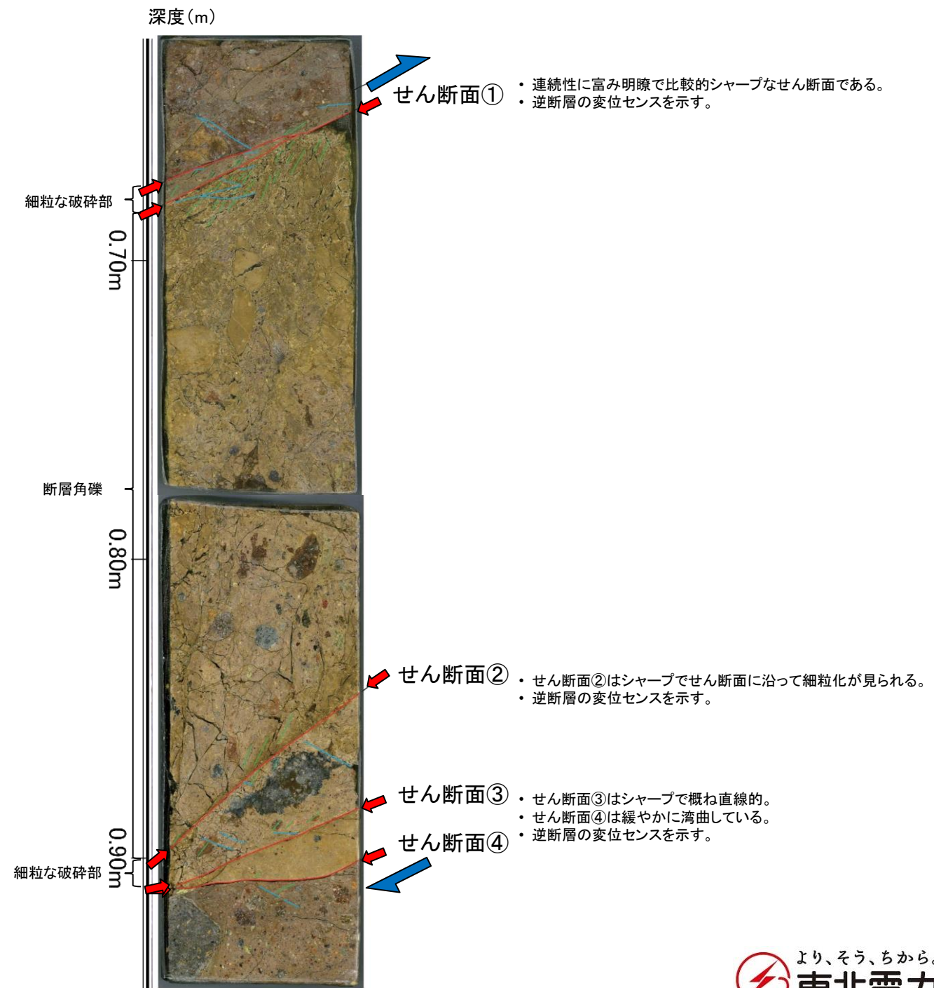
F-1断層破砕部研磨片画像
