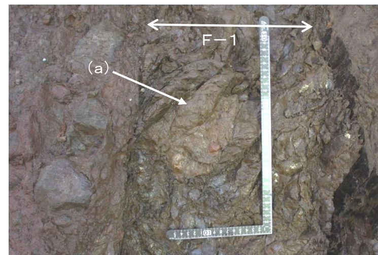
③弱破碎部は、割れ目に沿ってのみセピオライトが付着し、ブロック状にセピオライト化していない部分(a)を主とする。
