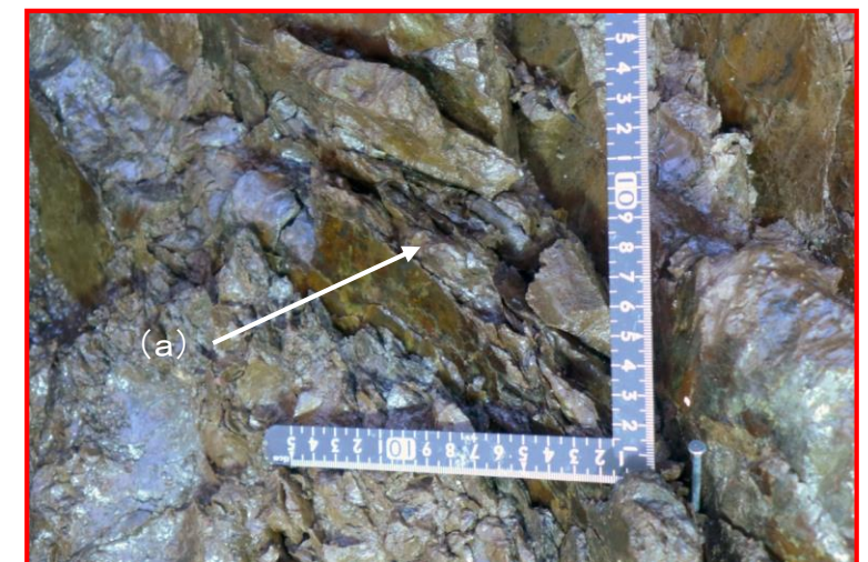
葉片状の岩片の表面にはセピオライトが認められる。葉片自体は硬質で、内部までセピオライトに置換される箇所(a)がある。
