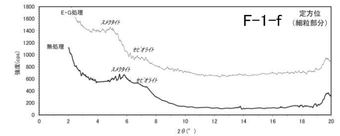
XRDチャート・上盤側葉片状部 変質鉱物はスメクタイトとセピオライト よくなる。
