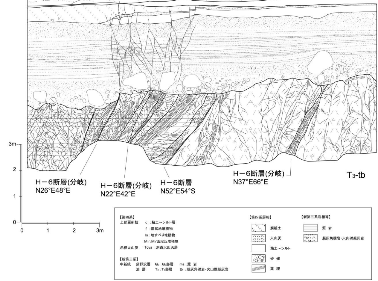
T6(2)トレンチ南面スケッチ
