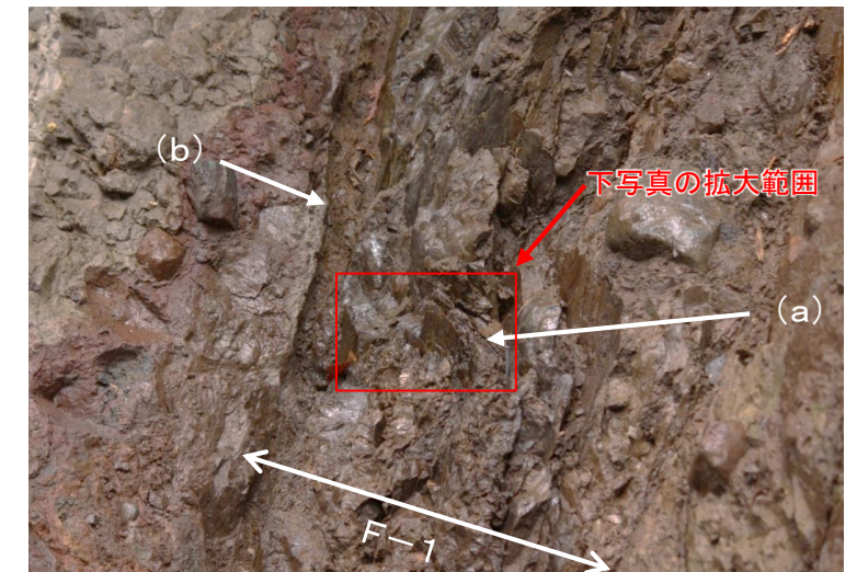
②葉片状破碎部では、湾曲した構造が認められ(a)全体的に硬質である。幅の狭い軟質部も認められるが(b), 下方で消滅することから、風化により軟質化したものと判断される。
