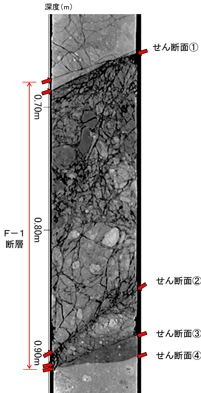
F-1断層破砕部X線CT画像(傾斜方向)
