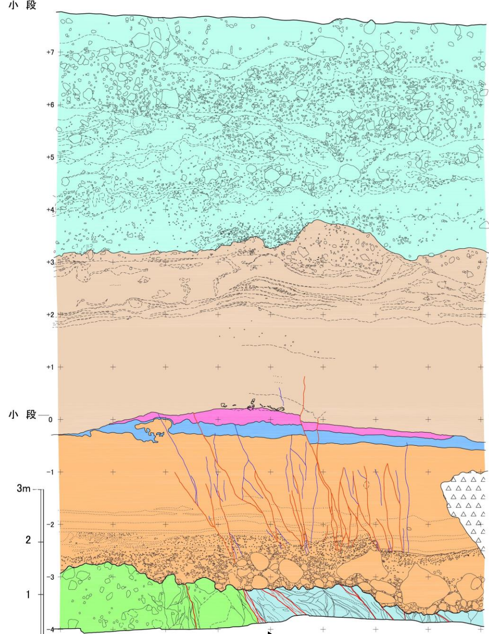
H-6断層 N29° E46° E
