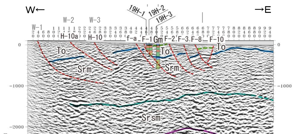
H28-Line3 マイグレーション深度断面(縦横比1:1)
