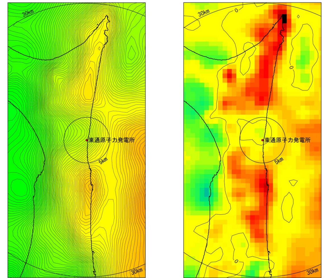
-75 -50 -25 0 25 50 75 100 125 150 175 mGal
