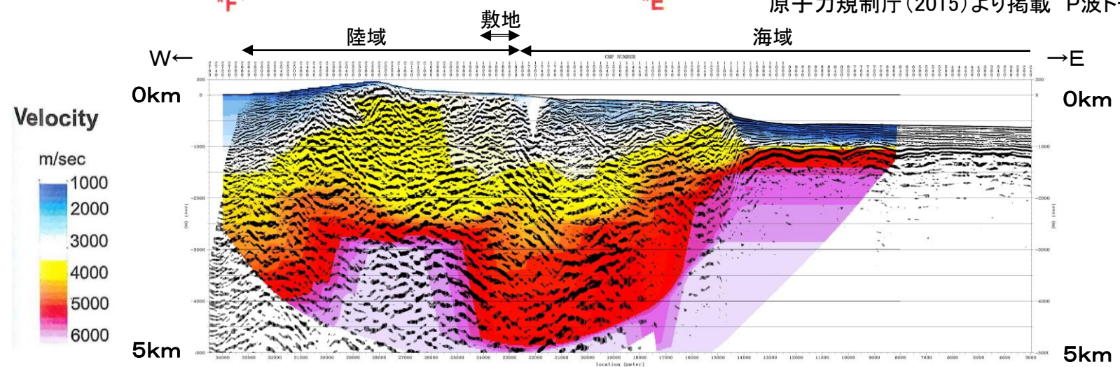
H24海陸統合探査 P波トモグラフィー解析結果
