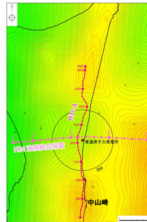
ブーゲー異常
