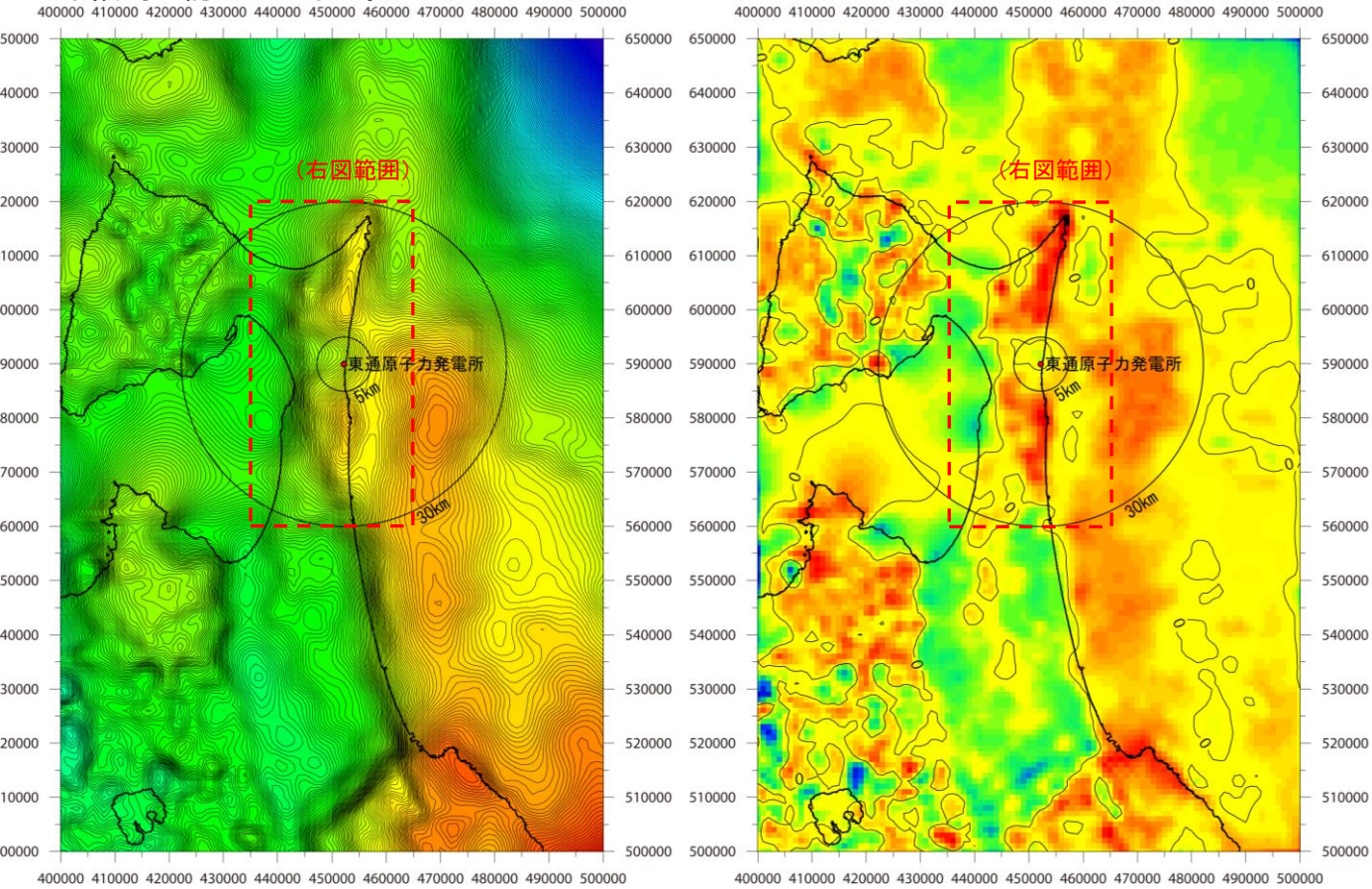
-75 -50 -25 0 25 50 75 100 125 150 175 mGal 仮定密度 \rho = 2.67\text{g/cm}^3 , 格子間隔1,000m, コンター間隔は1mGal
