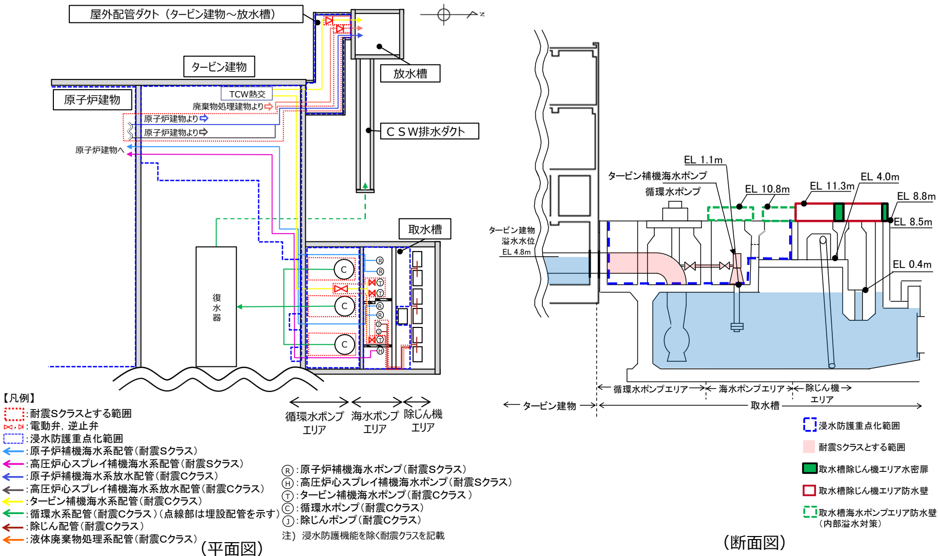
図 浸水防護重点化範囲内に設置する海域と接続する低耐震クラスの機器及び配管への対策
