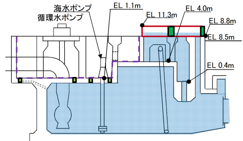
2号炉取水槽除じん機エリア防水壁及び水密扉 嵩上げ断面イメージ図
