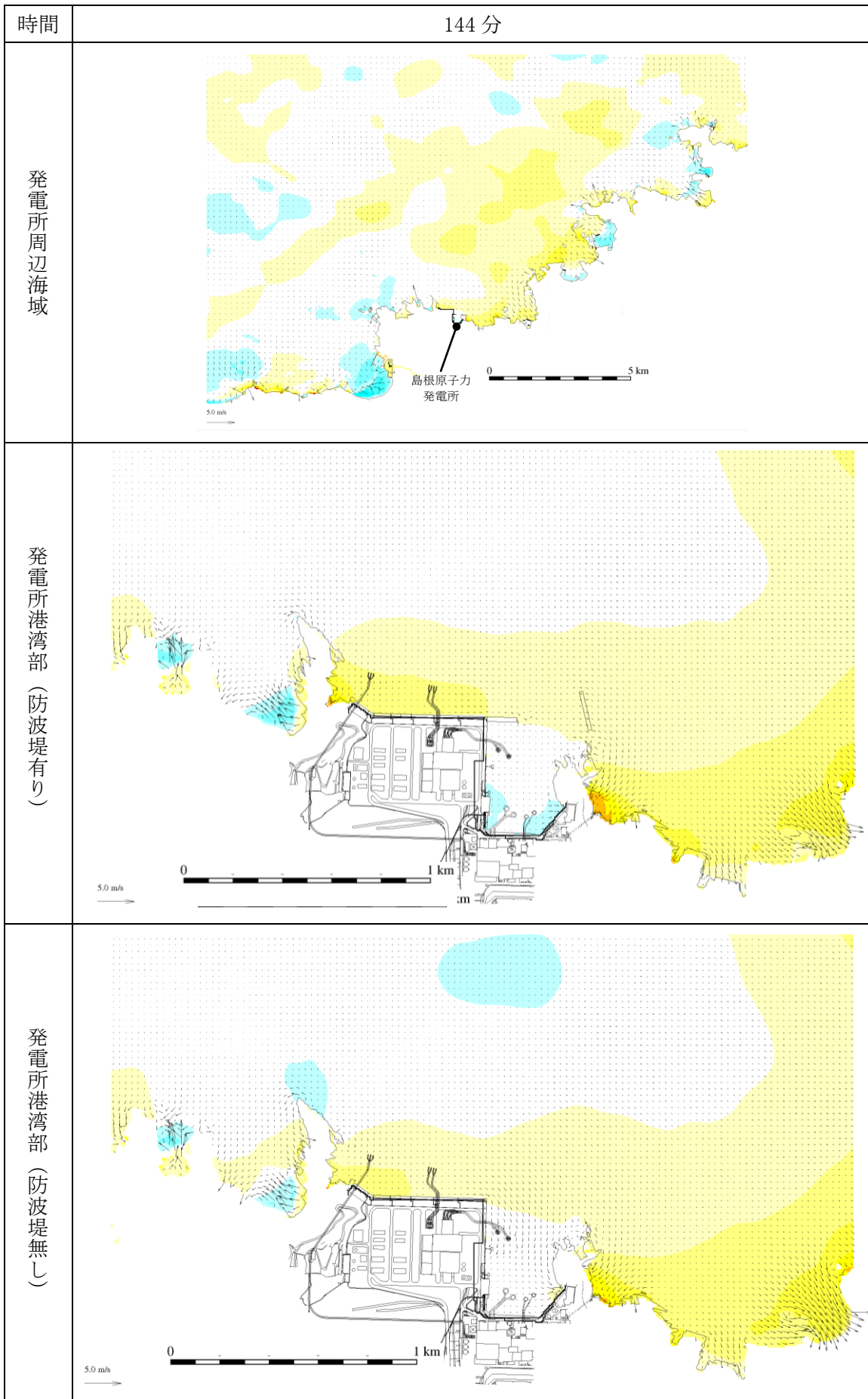
第 1 図(89) 基準津波 1 の水位変動・流向ベクトル
