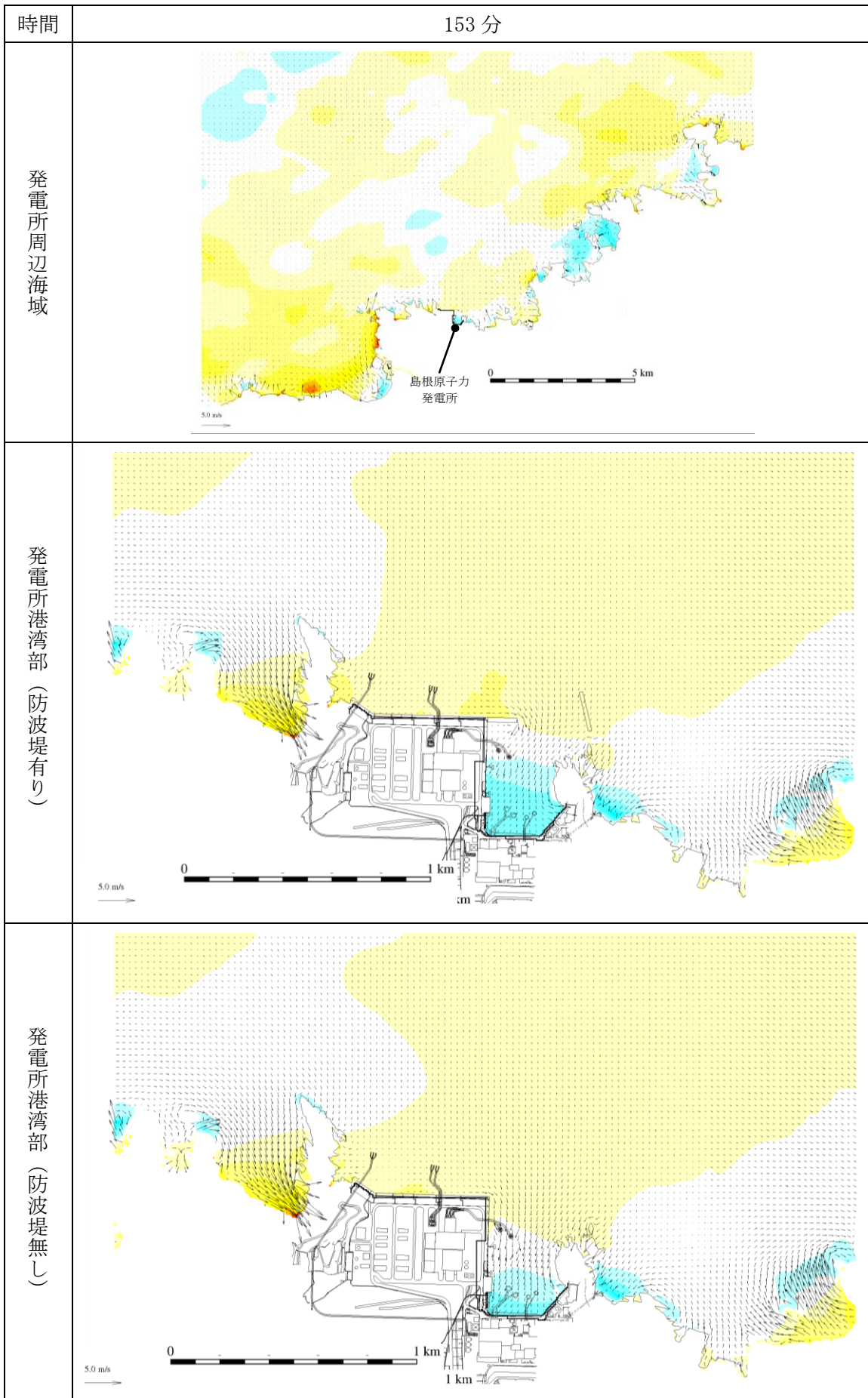
第 1 図(107) 基準津波 1 の水位変動・流向ベクトル
