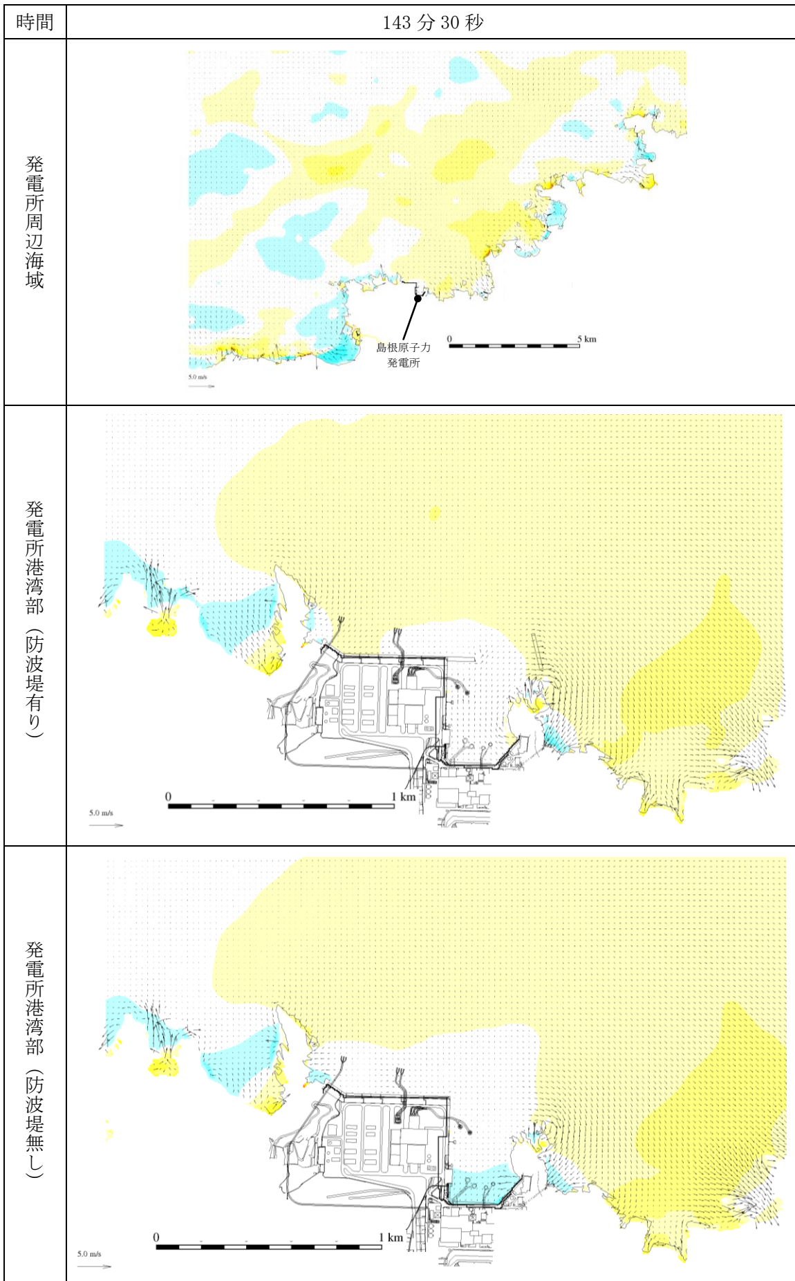
第 1 図(88) 基準津波 1 の水位変動・流向ベクトル
