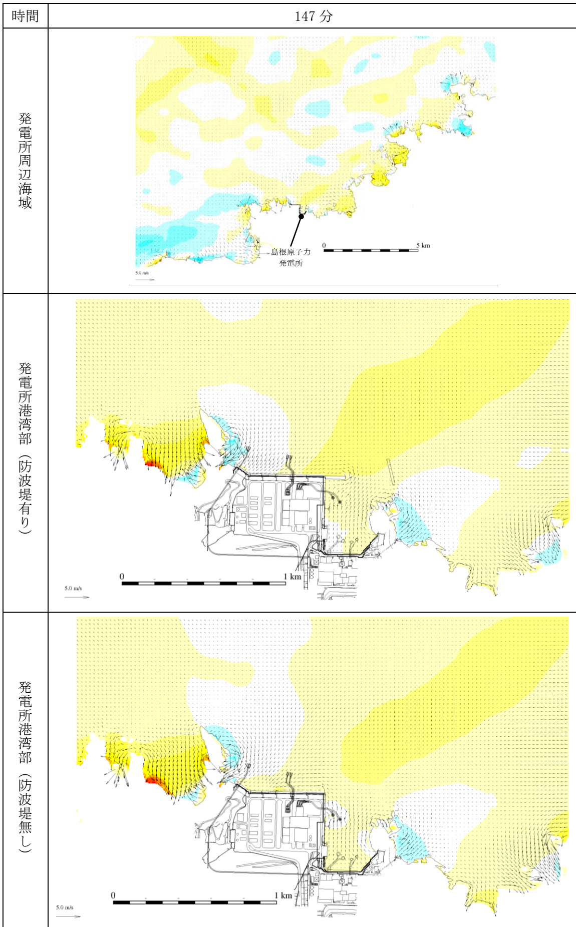
第 1 図(95) 基準津波 1 の水位変動・流向ベクトル
