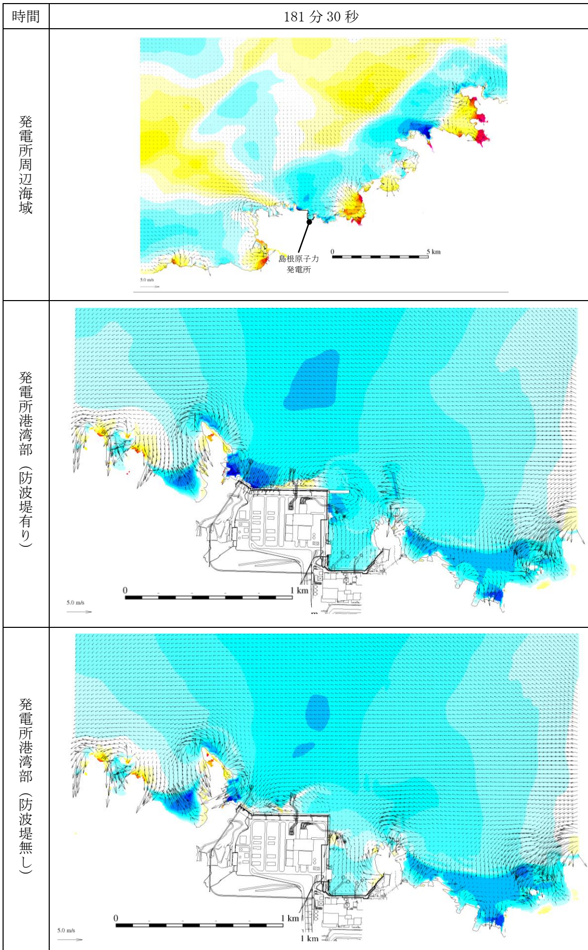
第 1 図(164) 基準津波 1 の水位変動・流向ベクトル
