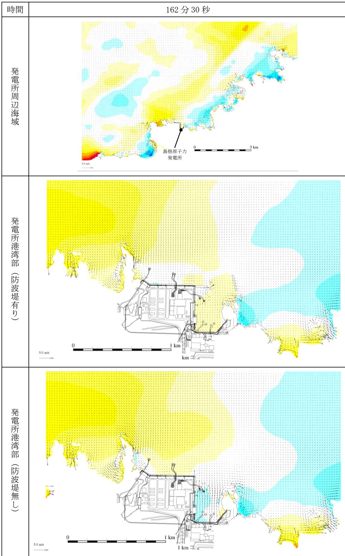
第 1 図(126) 基準津波 1 の水位変動・流向ベクトル
