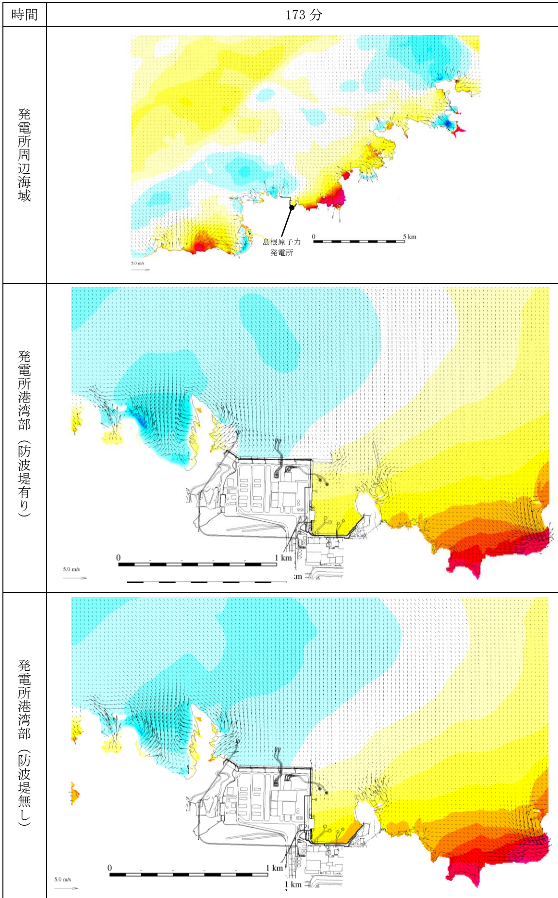
第 1 図(147) 基準津波 1 の水位変動・流向ベクトル
