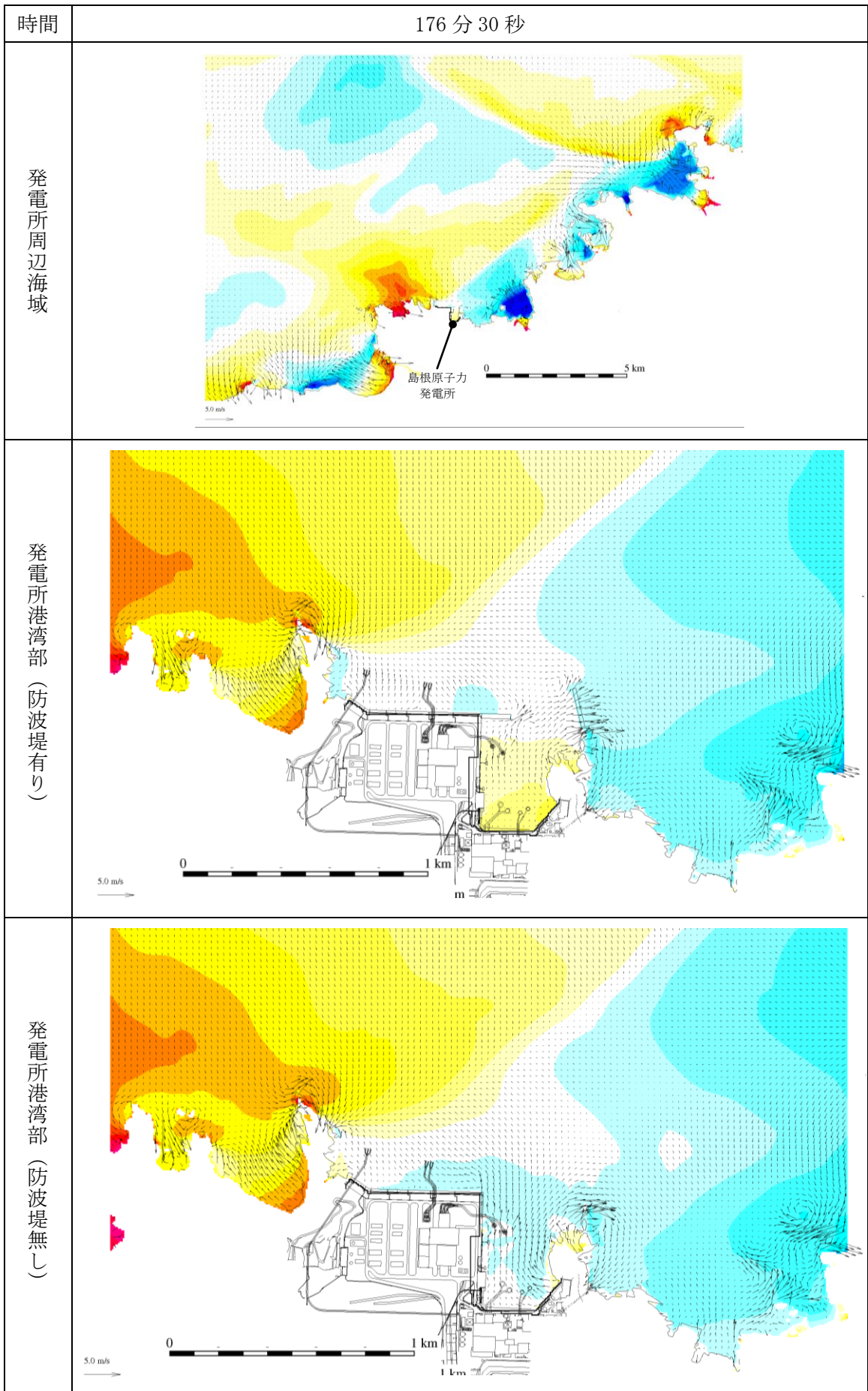
第 1 図 (154) 基準津波 1 の水位変動・流向ベクトル
