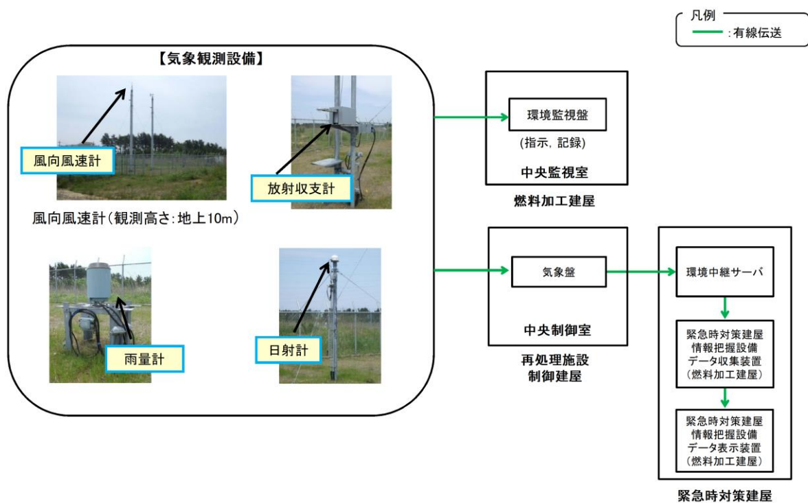
第9. 1. 1図 気象観測設備の外観及び伝送概略図
