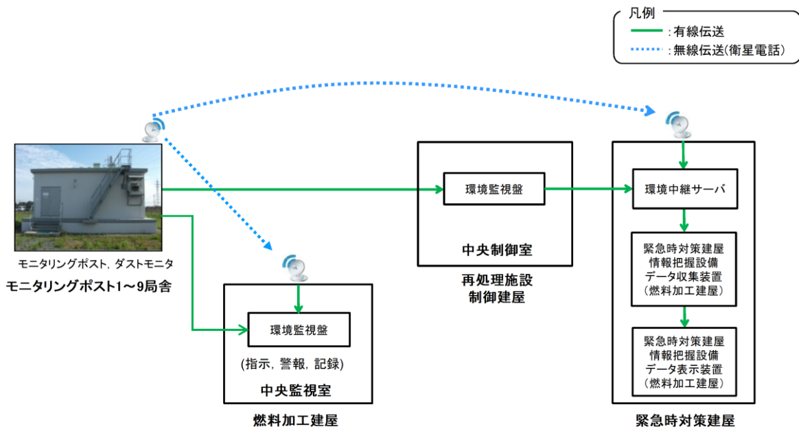
第3. 1. 3図 モニタリングポスト等の系統概要図
