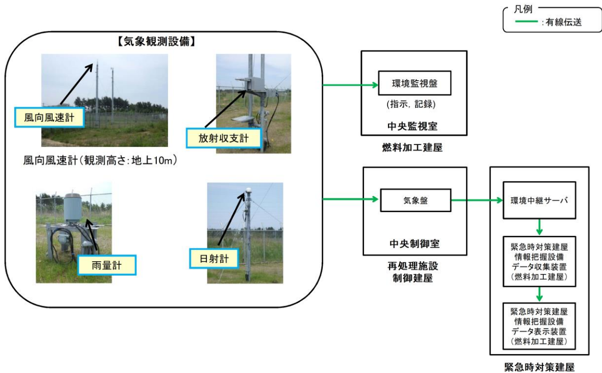
第 6 図 気象観測設備の外観及び伝送概略図
