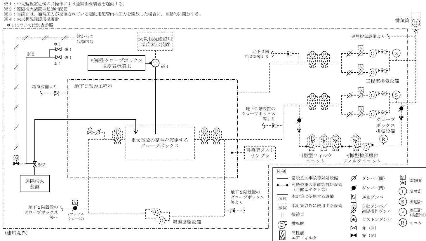
第 2-3.1 図 代替消火設備及び代替火災感知設備の系統概要図 (外的事象の対処時)
