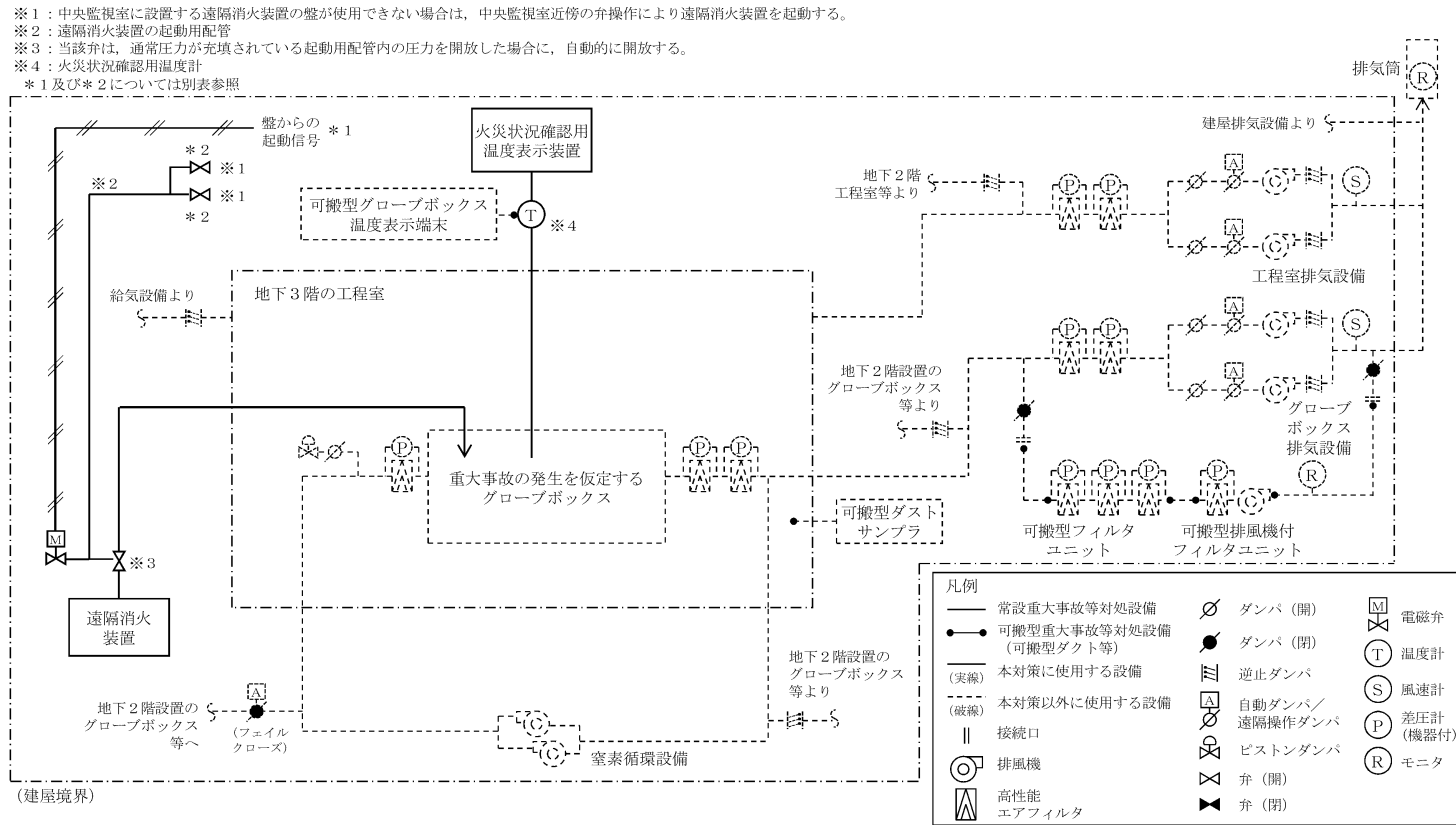
第 2-3.2 図 代替消火設備及び代替火災感知設備の系統概要図 (内的事象の対処時)
