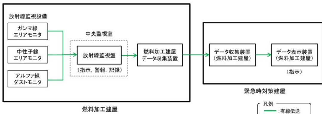
第1図 エリアモニタ及びダストモニタの系統概要図
