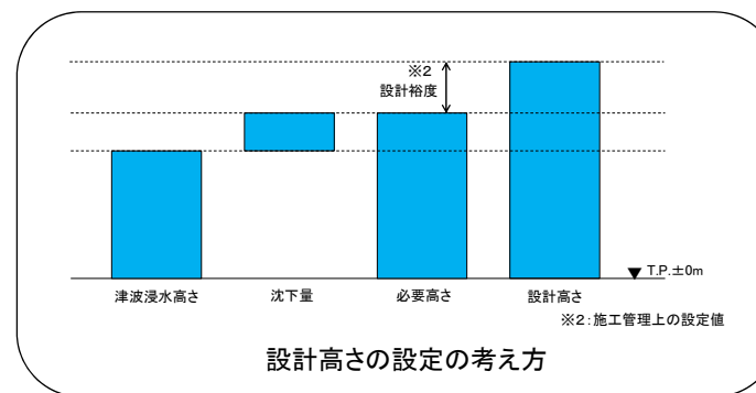
設計高さと津波浸水高さの関係
