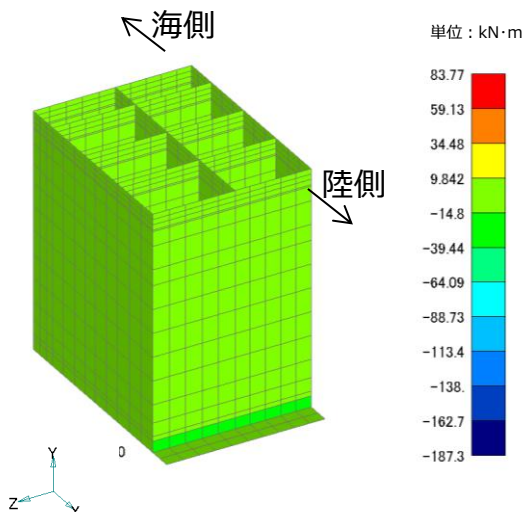
曲げモーメントコンター図(鉛直方向)
