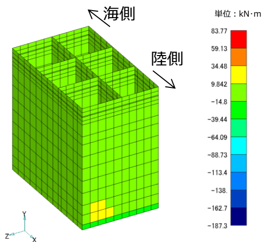
曲げモーメントコンター図(鉛直方向)
