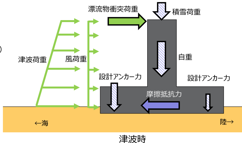
滑動の照査における荷重イメージ
