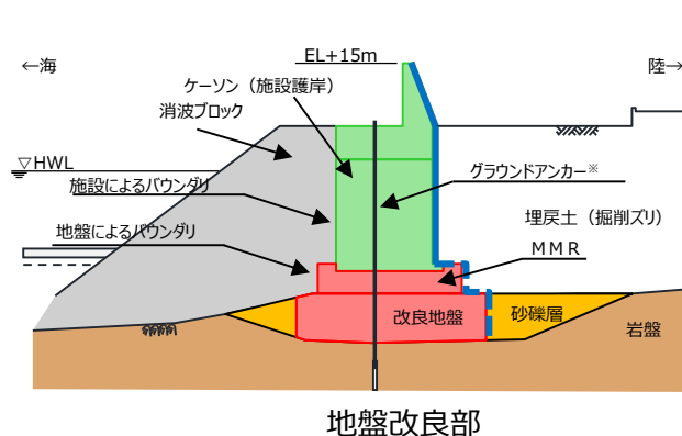
波返重力擁壁（改良地盤部）の「施設」・「地盤」の範囲
