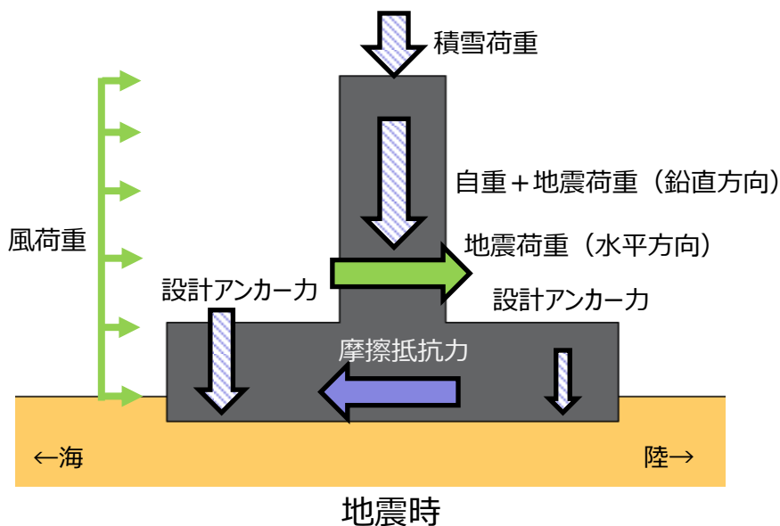
滑動の照査における荷重イメージ
