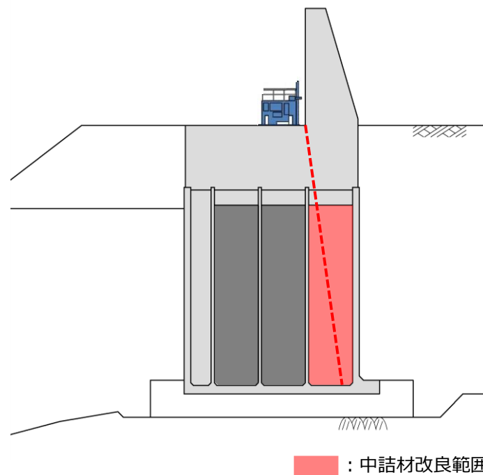
ケーソン中詰材改良の施工イメージ
