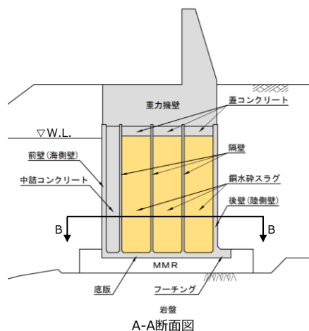
(ケーソン部材名称)
