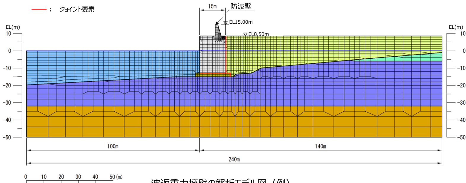
波返重力擁壁の解析モデル図（例）
