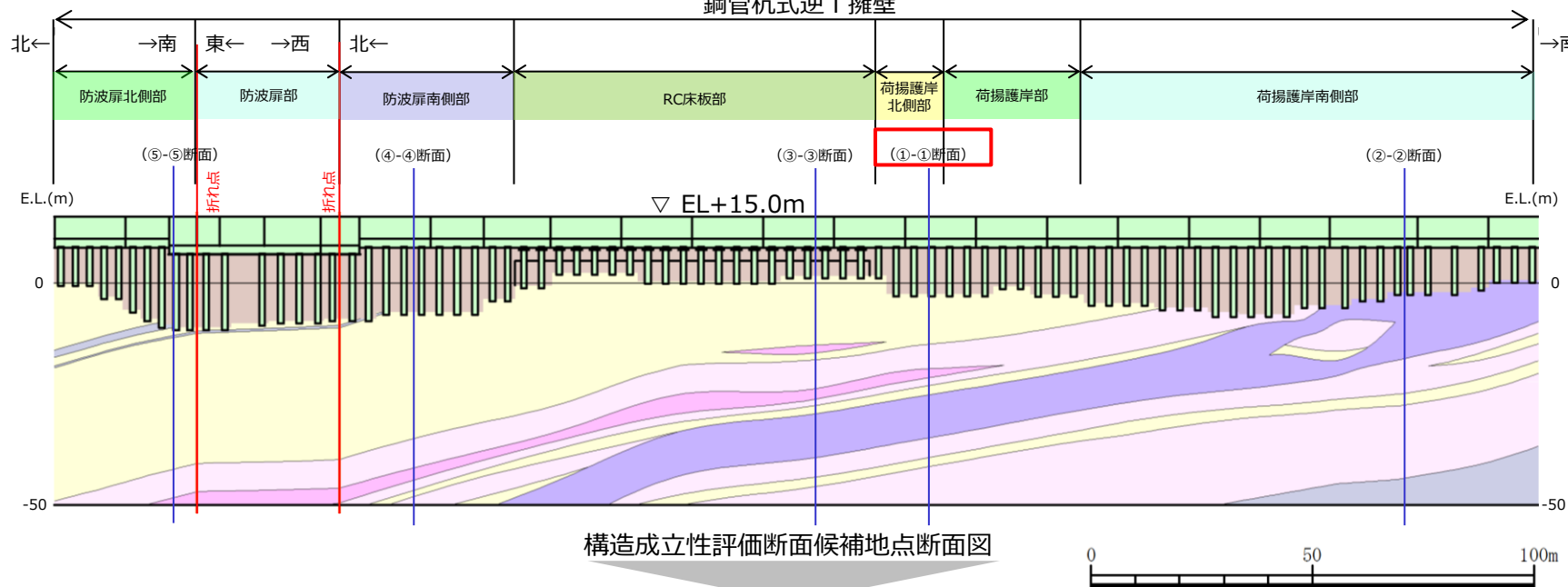
鋼管杭式逆T擁壁
