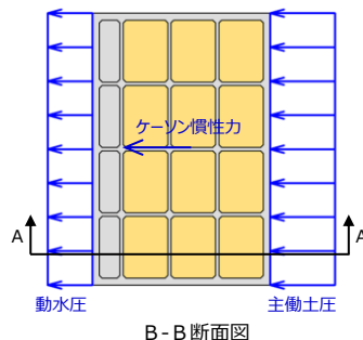
ケーソンに作用する荷重図
