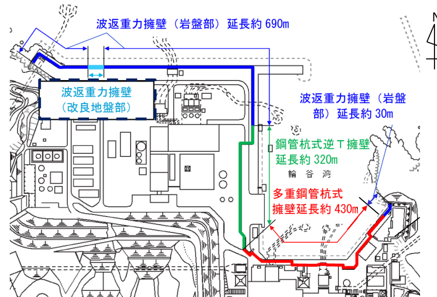
防波壁の位置図
