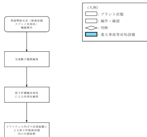
第 1.6-29 図 重大事故等時の対応手段選択フローチャート
