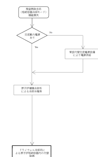
第 1.6-30 図 重大事故等時の対応手段選択フローチャート
