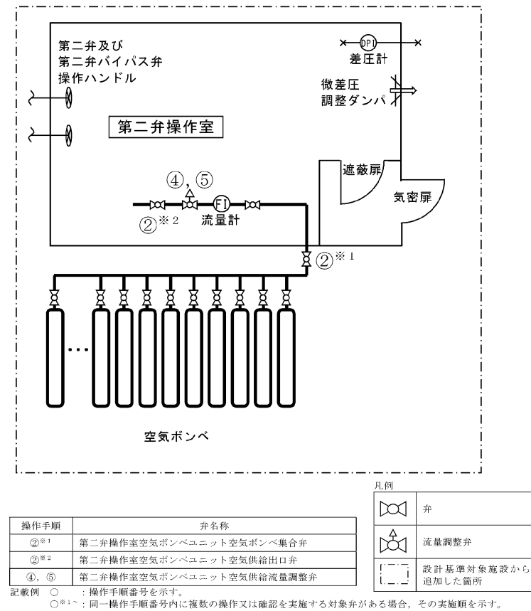
第 1.7-6 図 第二弁操作室の正圧化 概要図
