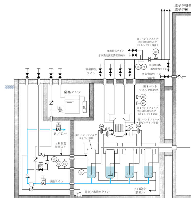
図 4.2.4-1 スクラビング水移送時の系統状態概要図
