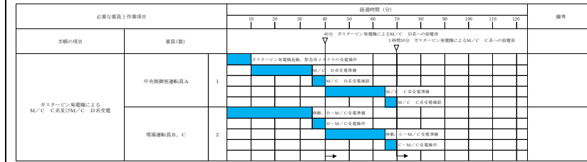
第 3.14-19 図 ガスタービン発電機によるM/C受電のタイムチャート
