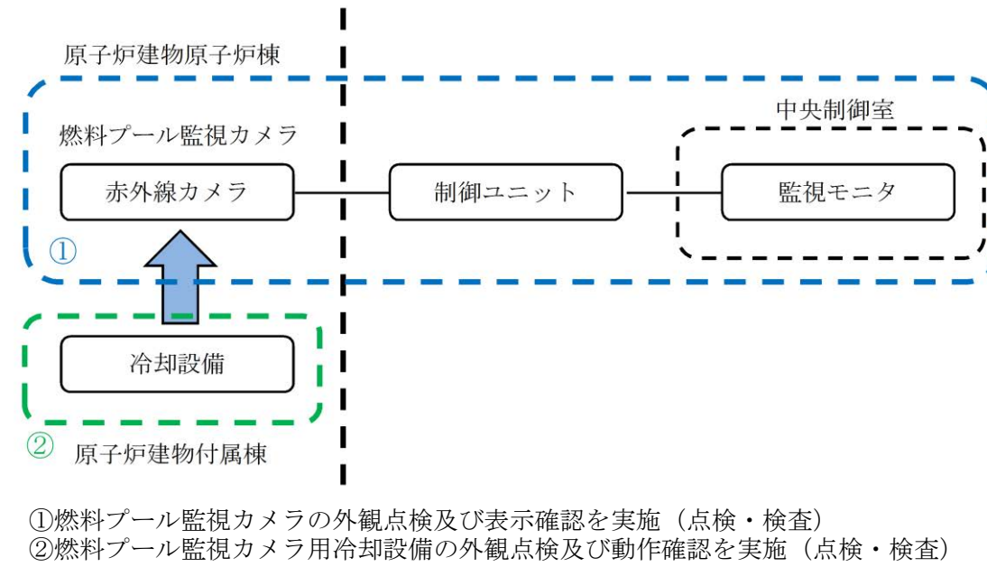
第 58-5-14 図 燃料プール監視カメラ (SA) 及び燃料プール監視カメラ用冷却設備の試験及び検査
