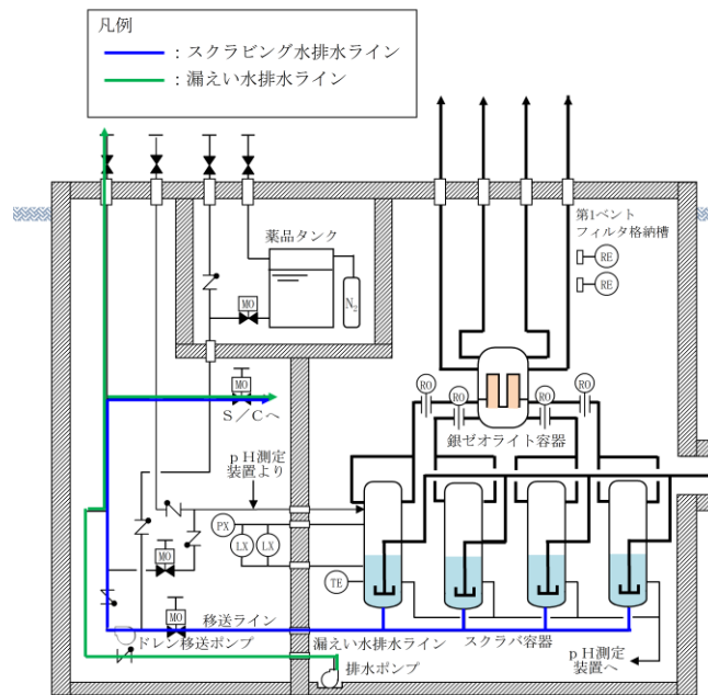
図12 排水設備 系統概略図（補給時）
