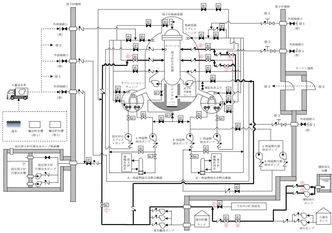
図2 消火系（消火ポンプ使用）による炉心注水 概略系統図
