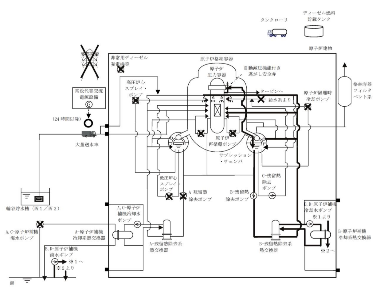
第 2. 3. 1. 1-1(3) 図 「全交流動力電源喪失（外部電源喪失+DG失敗）+HPCS失敗」の重大事故等対策の概略系統図（原子炉注水及び原子炉格納容器除熱）
