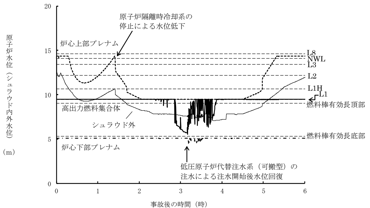
図6 操作開始時間 50 分遅れのケースにおける原子炉水位 (シユラウド内外水位) の推移
