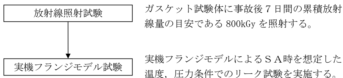
図1 実機フランジ模擬試験の試験フロー
