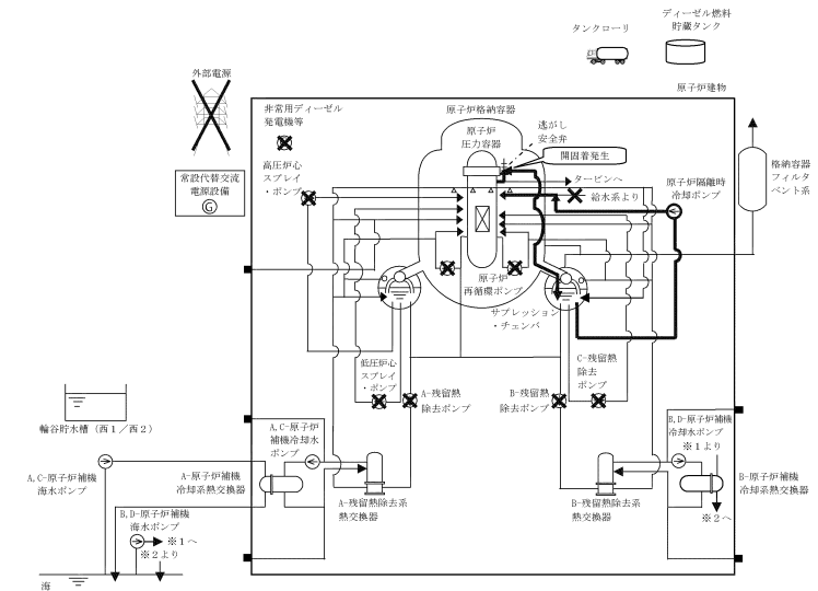
第 2.3.4.1-1(1) 図 「全交流動力電源喪失 (外部電源喪失+DG 失敗)+SRV 再閉失敗+HPCS 失敗」の重大事故等対策の概略系統図 (原子炉注水)
