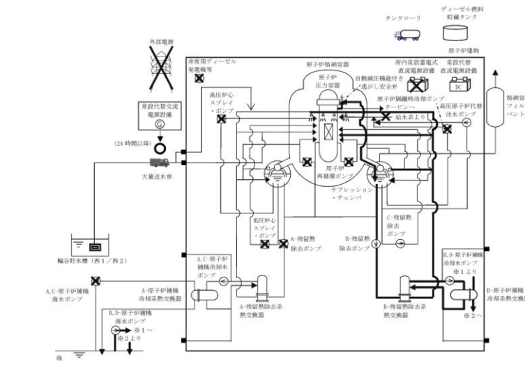
第 2.3.3.1-1(3) 図 「全交流動力電源喪失 (外部電源喪失+DG 失敗) +直流電源喪失」の重大事故等対策の概略系統図 (原子炉注水及び原子炉格納容器除熱)
