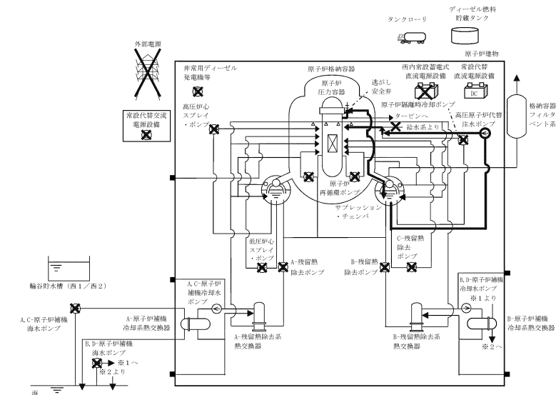
第 2.3.3.1-1(1) 図 「全交流動力電源喪失 (外部電源喪失+DG 失敗) + 直流電源喪失」の重大事故等対策の概略系統図 (原子炉注水)
