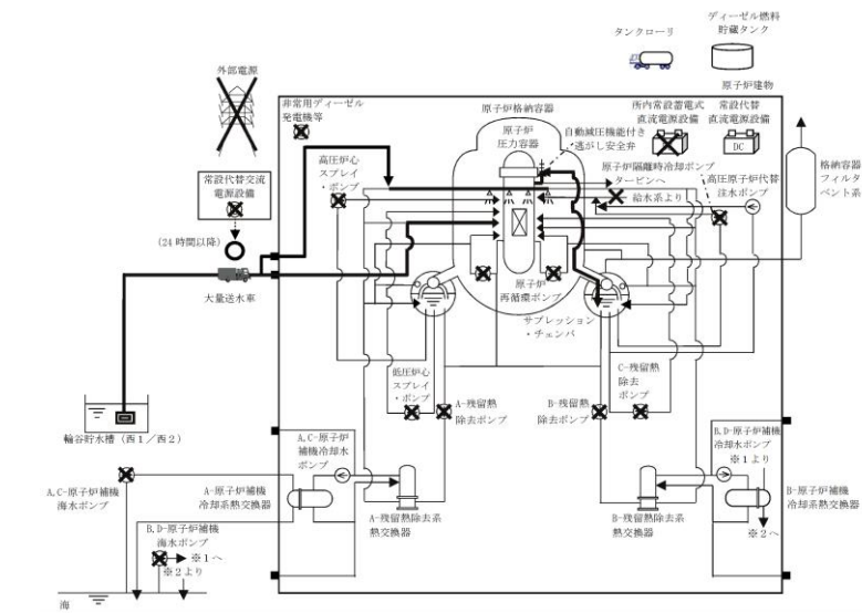
第 2.3.3.1-1(2) 図 「全交流動力電源喪失 (外部電源喪失+DG 失敗) + 直流電源喪失」の重大事故等対策の概略系統図 (原子炉減圧, 原子炉注水及び原子炉格納容器冷却)
