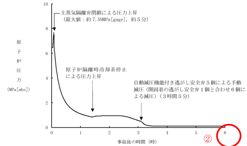
第2.3.4.3-1(1) 図 操作開始時間45分遅れのケースにおける原子炉圧力の推移
