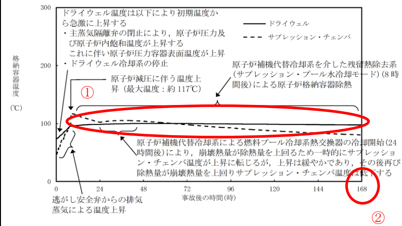
第 2. 4. 1. 2-1(11) 図 格納容器温度の推移
