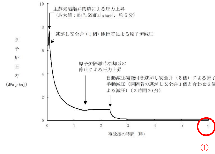
第 2.3.4.2-1(1) 図 原子炉圧力の推移
