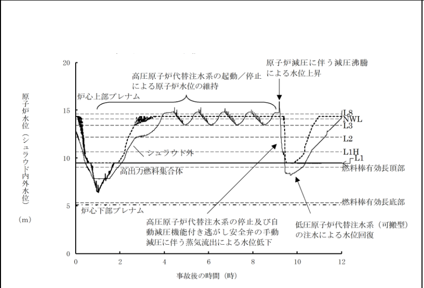
第 2.3.2.3-1(2) 図 事象発生 60 分後に注水を開始したケースにおける原子炉水位 (シユラウド内外水位) の推移
