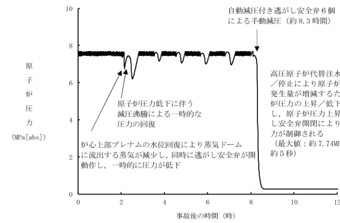
第 2.3.2.2-1(1) 図 原子炉圧力の推移
