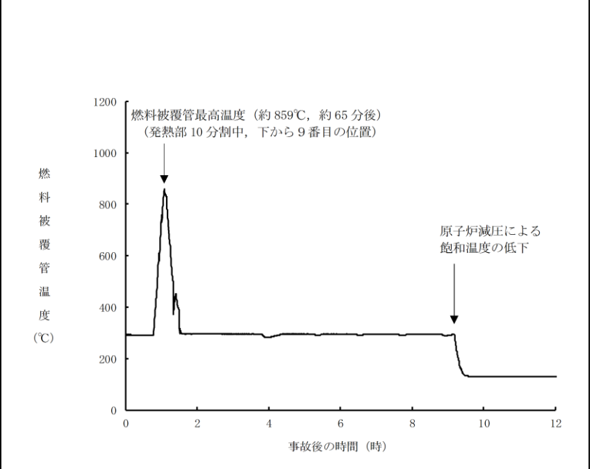
第 2.3.2.3-1(3) 図 事象発生 60 分後に注水を開始したケースにおける燃料被覆管温度の推移
