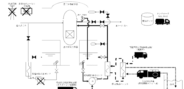
第 2.3.1.4 図 「全交流動力電源喪失 (外部電源喪失+DG 喪失)」 の重大事故等対策の概略系統図 (4/4) (原子炉注水及び原子炉格納容器除熱)
