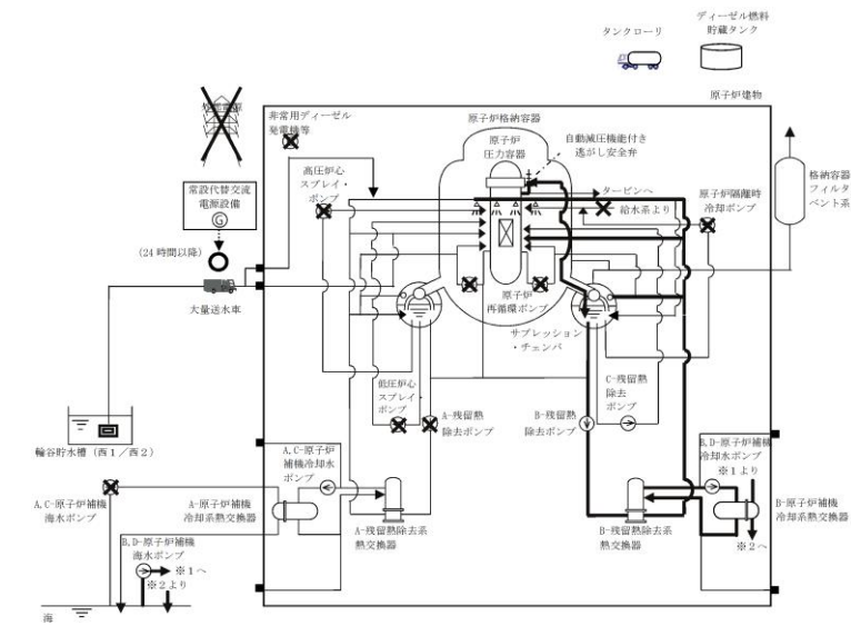
第 2.3.1.1-1(3) 図 「全交流動力電源喪失 (外部電源喪失+ DG失敗) +HPCS失敗」の重大事故等対策の概略系統図 (原子炉注水及び原子炉格納容器除熱)
