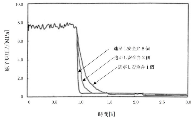
第1図 原子炉減圧時の原子炉圧力の推移
