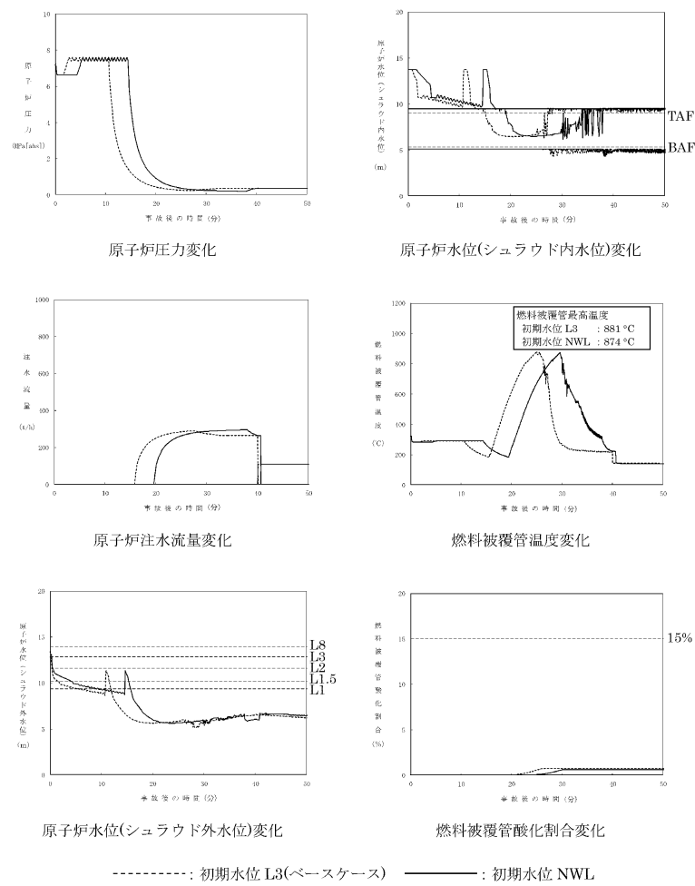
第2図 原子炉初期水位に関する感度解析 (K7, ADS(L1)+MUWC 2 台作動)
