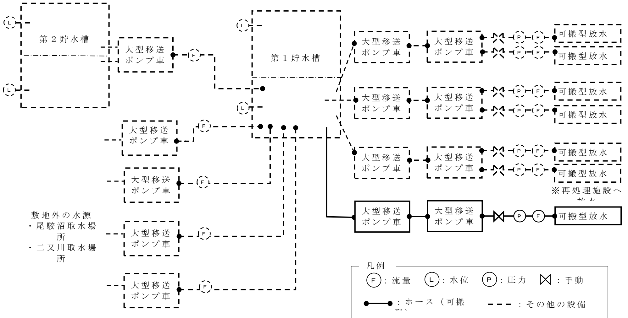
第3図 工場等外への放射性物質の拡散を抑制するための設備の系統概要図 (その1)
