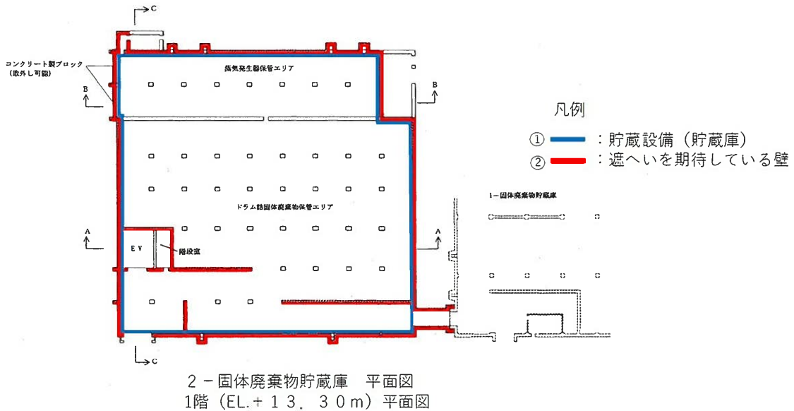
第2図 既設置許可の2 - 固体廃棄物貯蔵庫 (貯蔵庫及び遮へいの部分の区別)
