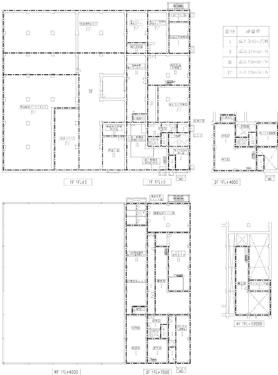
第 30-3 図 廃棄物搬出建屋の線量率区分(1/2)
