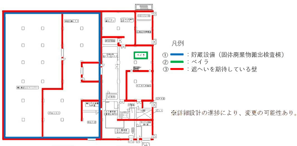
廃棄物搬出建屋 平面図 1階 (EL. + 17.00 m) 平面図
