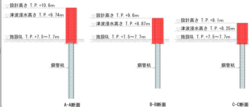
設計高さ(設計高さ)の関係
