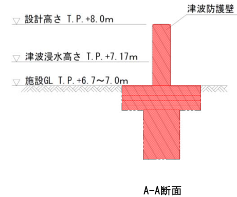
A-A断面 設計高さと津波浸水高さの関係
