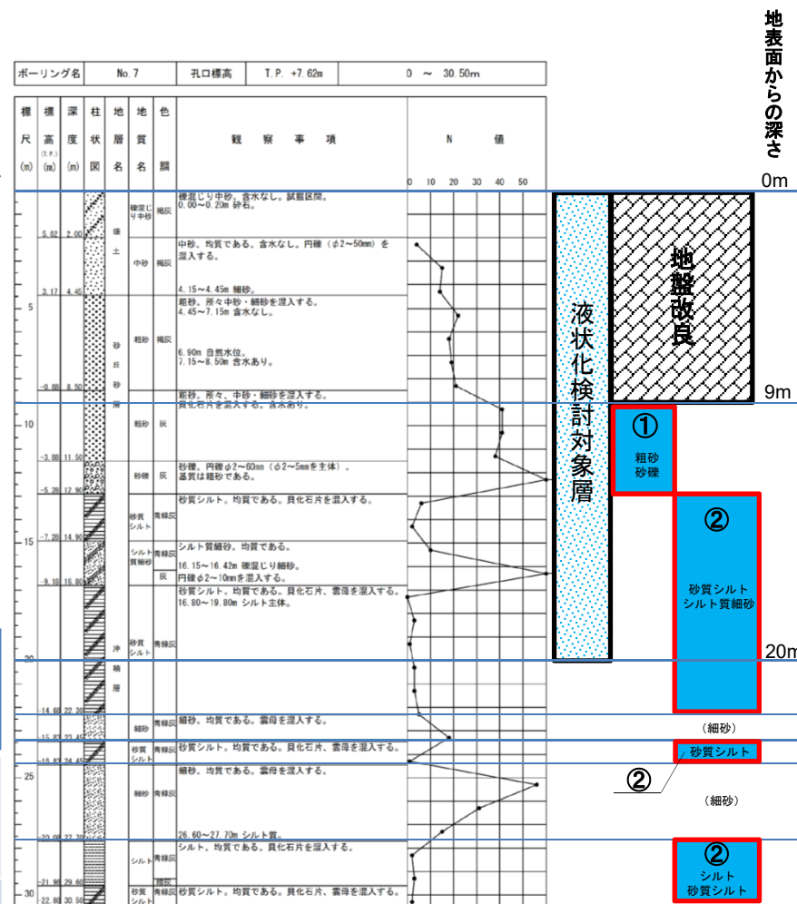
図 1-1-5-1.10 ボーリング柱状図(第2保管廃棄施設 No.7)
