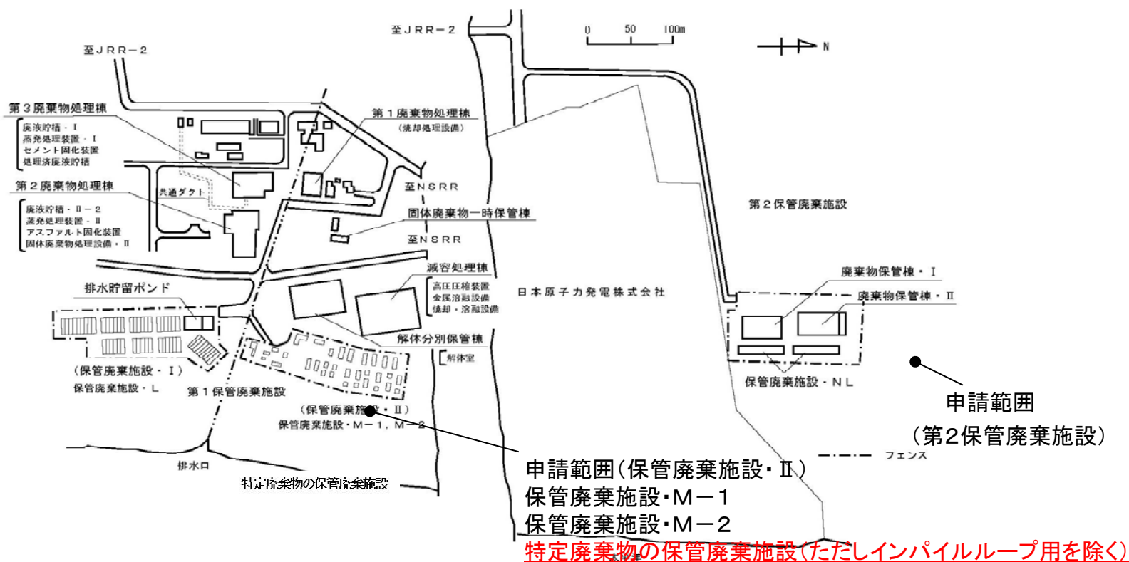
第4図 放射性廃棄物処理場配置図
