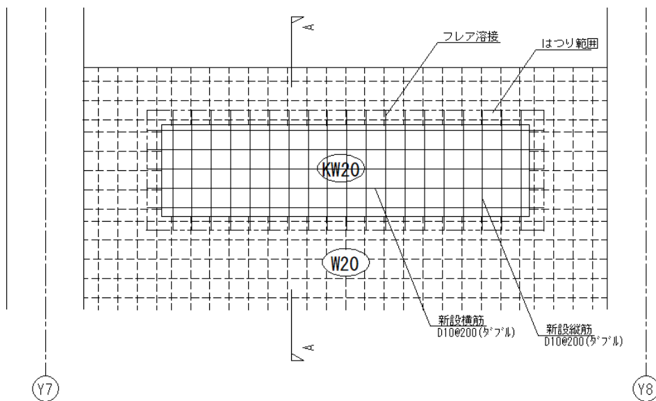
〔側面配筋図〕
