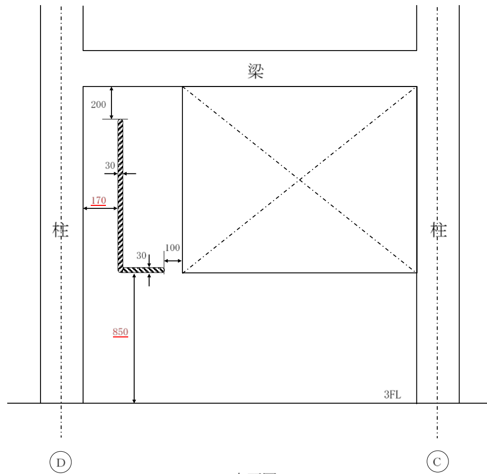
立面図 [単位: mm]
