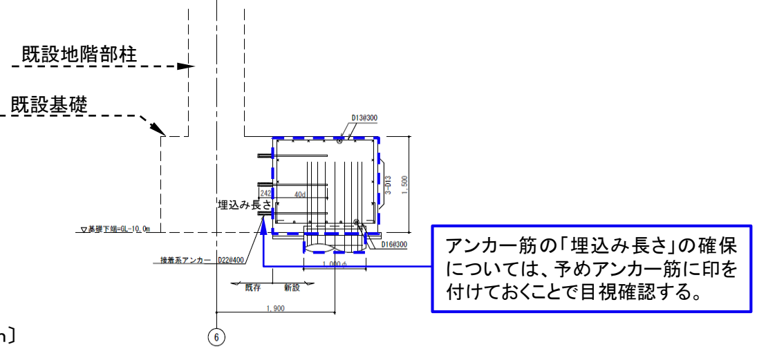
〔断面配筋図〕
