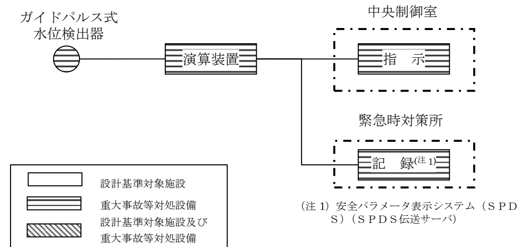
図17 燃料プール水位 (SA) の概略構成図
