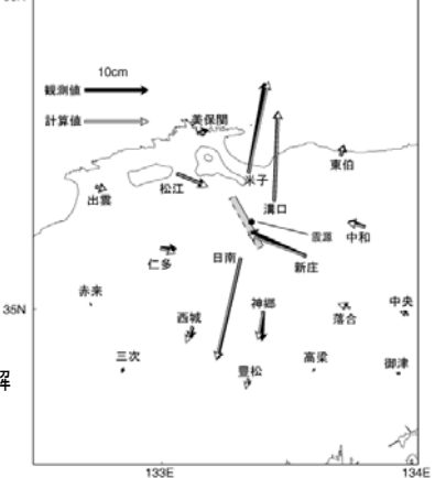
断層パラメーター 断層北西端の位置 東経133度18分 北緯35度21分 上板の深さ 1km 断層の長さ 20km (長さ) x 10km (幅) 歪角 北から時計回りに152度 傾斜角: 86度 すべり角: -7度 すべり量: 1.4m 補正係数: 0.6倍角: 6.6倍角 国土地理院(2000)より抜粋
