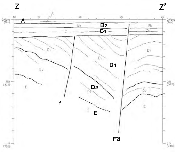
Z-Z' 断面
