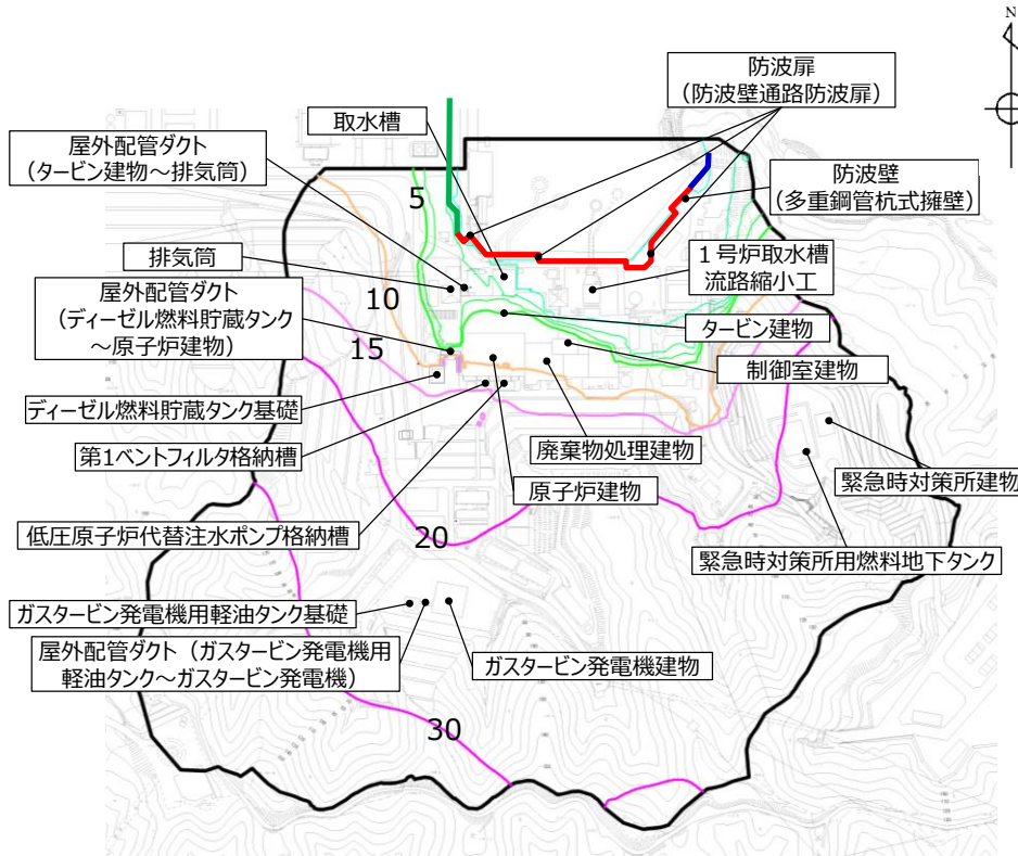
1, 2号炉エリア
