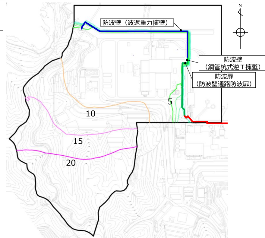
3号炉エリア
