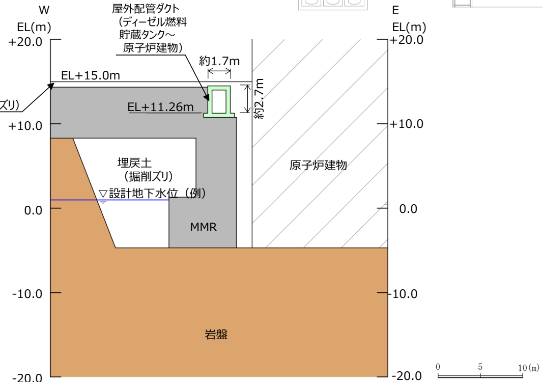
屋外配管ダクト（ディーゼル燃料貯蔵タンク～原子炉建物） ②－②断面図
