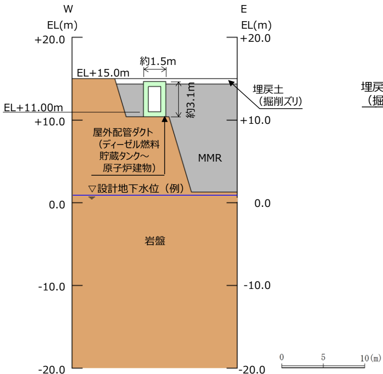
屋外配管ダクト（ディーゼル燃料貯蔵タンク～原子炉建物） ①－①断面図
