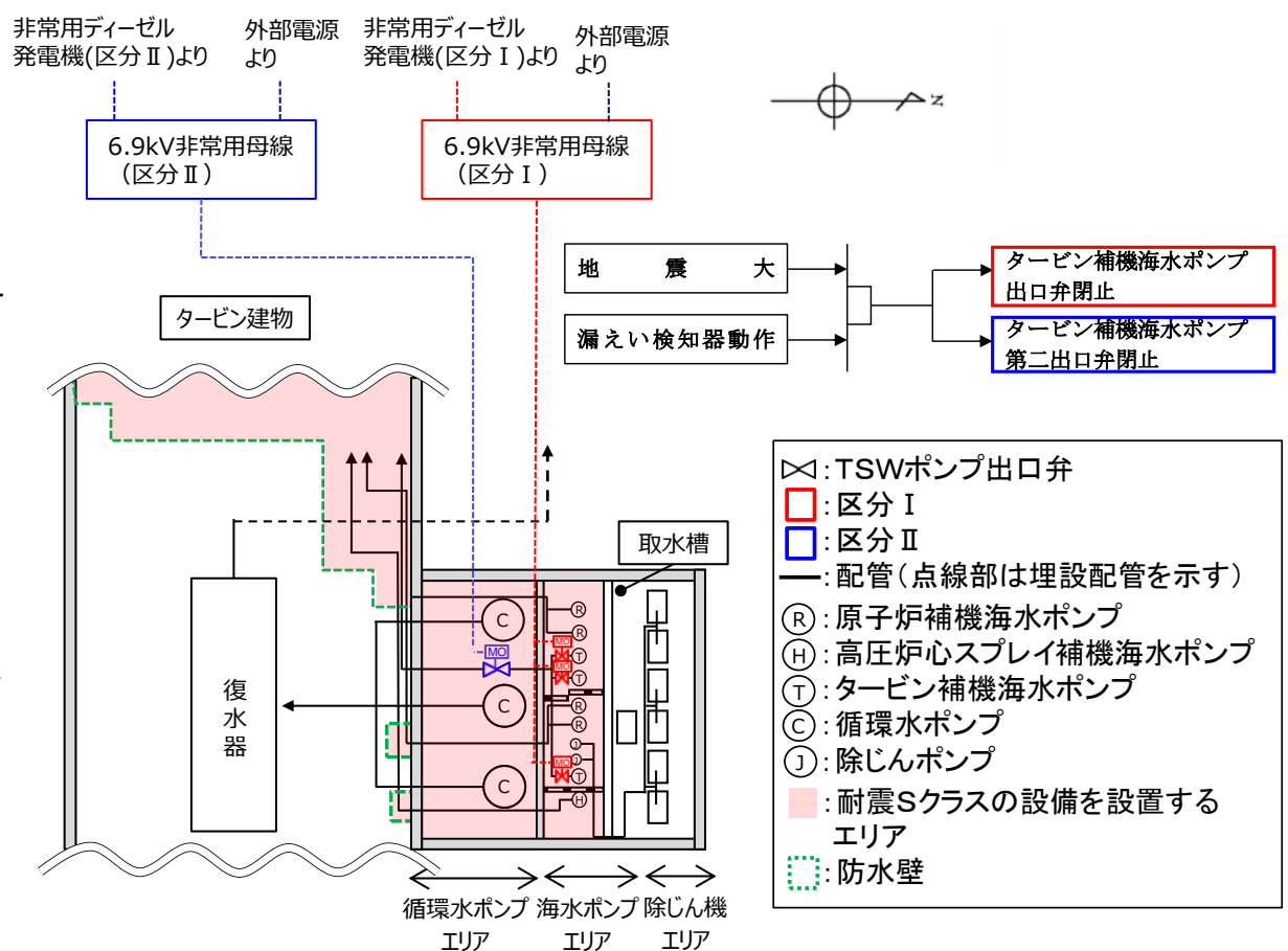
図1 タービン補機海水ポンプ出口弁設置概要図
