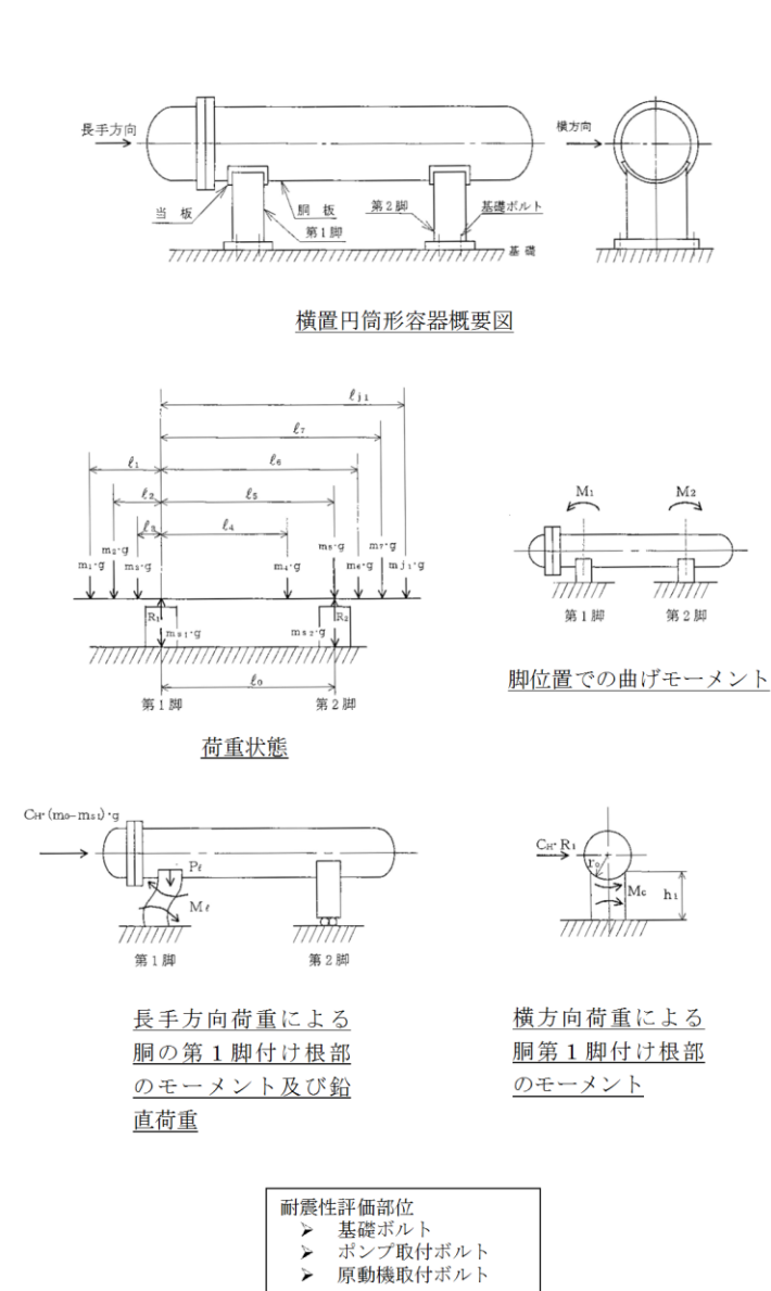
図7-2 耐震評価の概要 (横置円筒形容器の例)
