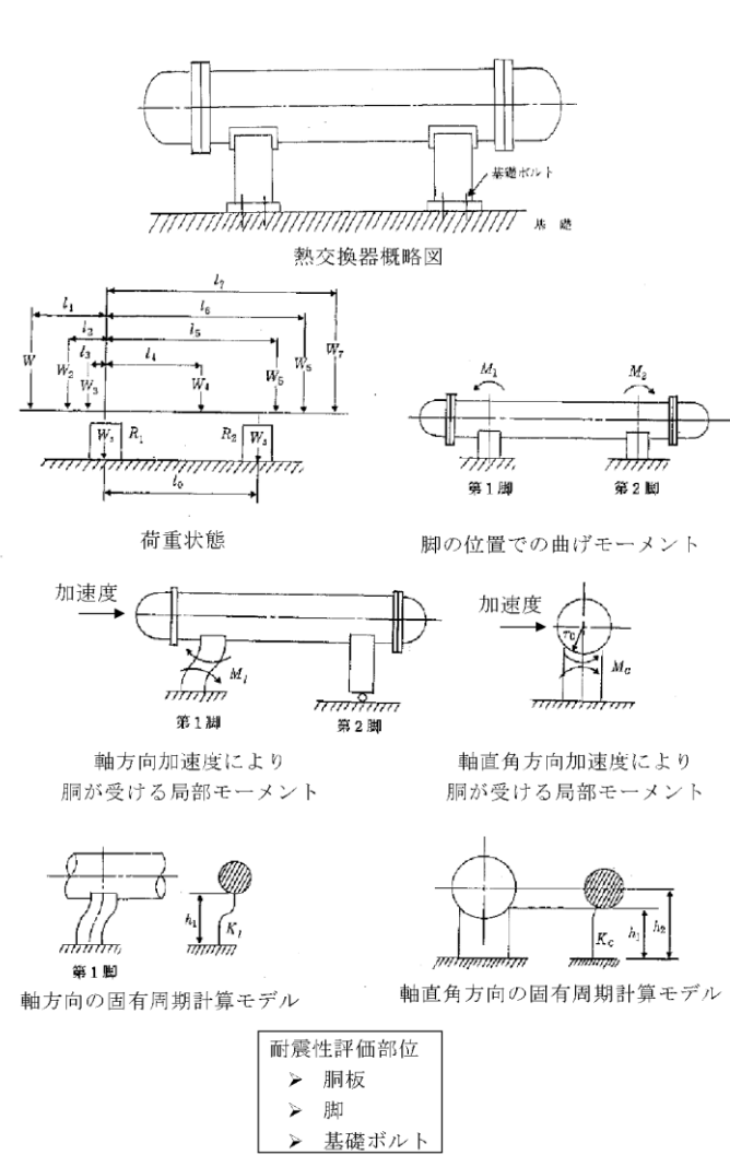
第7.3.1-2 図 耐震評価の概要 (横置円筒形容器の例)
