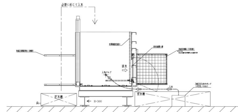
図 3-3 溢水通水扉通水試験装置概要図
