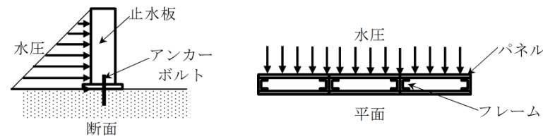
第8図(1/2) 強度評価概要図
