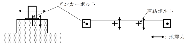
第8図(2/2) 耐震評価概要図
