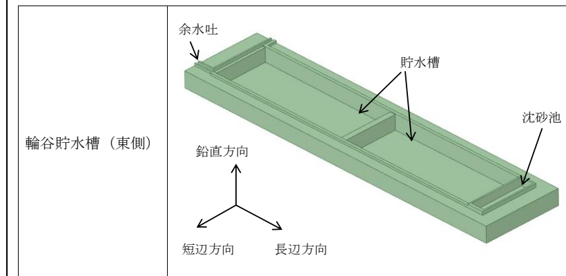
図2 解析モデル図
