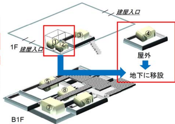
第1図 地下に移設する薬品タンク
