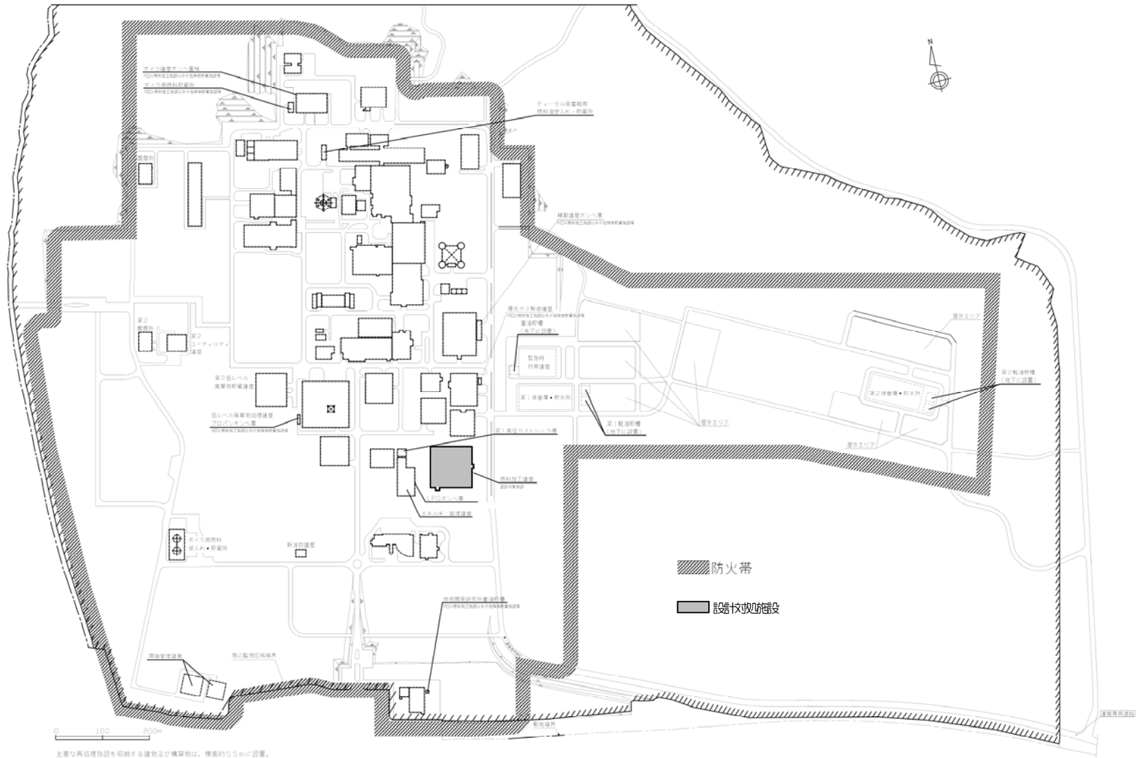
第3図 設計対処施設の配置図
