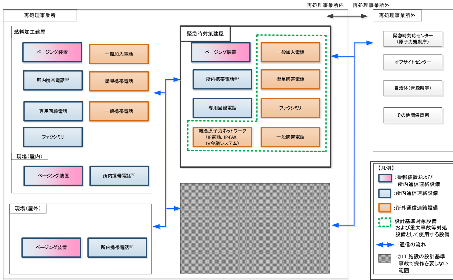
第 2 . 1 . 5 - 1 図 再処理事業所内外の通信設備の概要図
