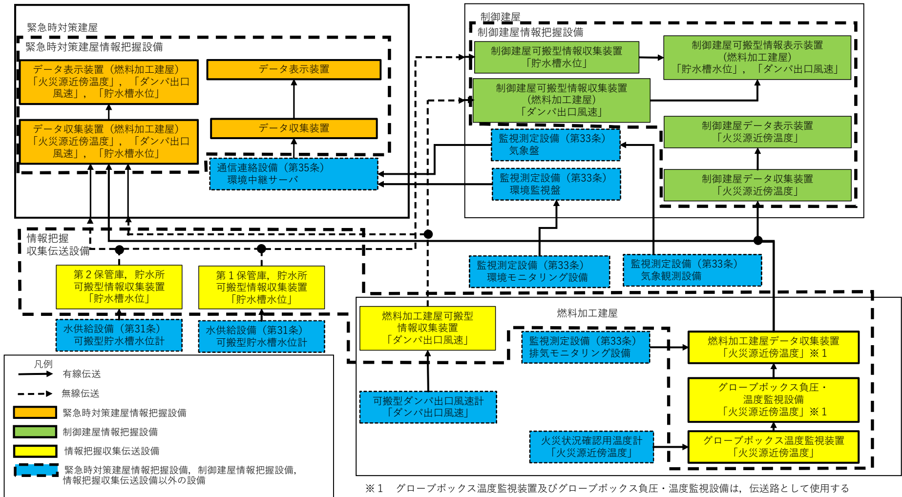
第3-18-1 図 情報把握設備 系統概要図 (重大事故等が発生し、全交流電源の喪失を伴わない場合)
