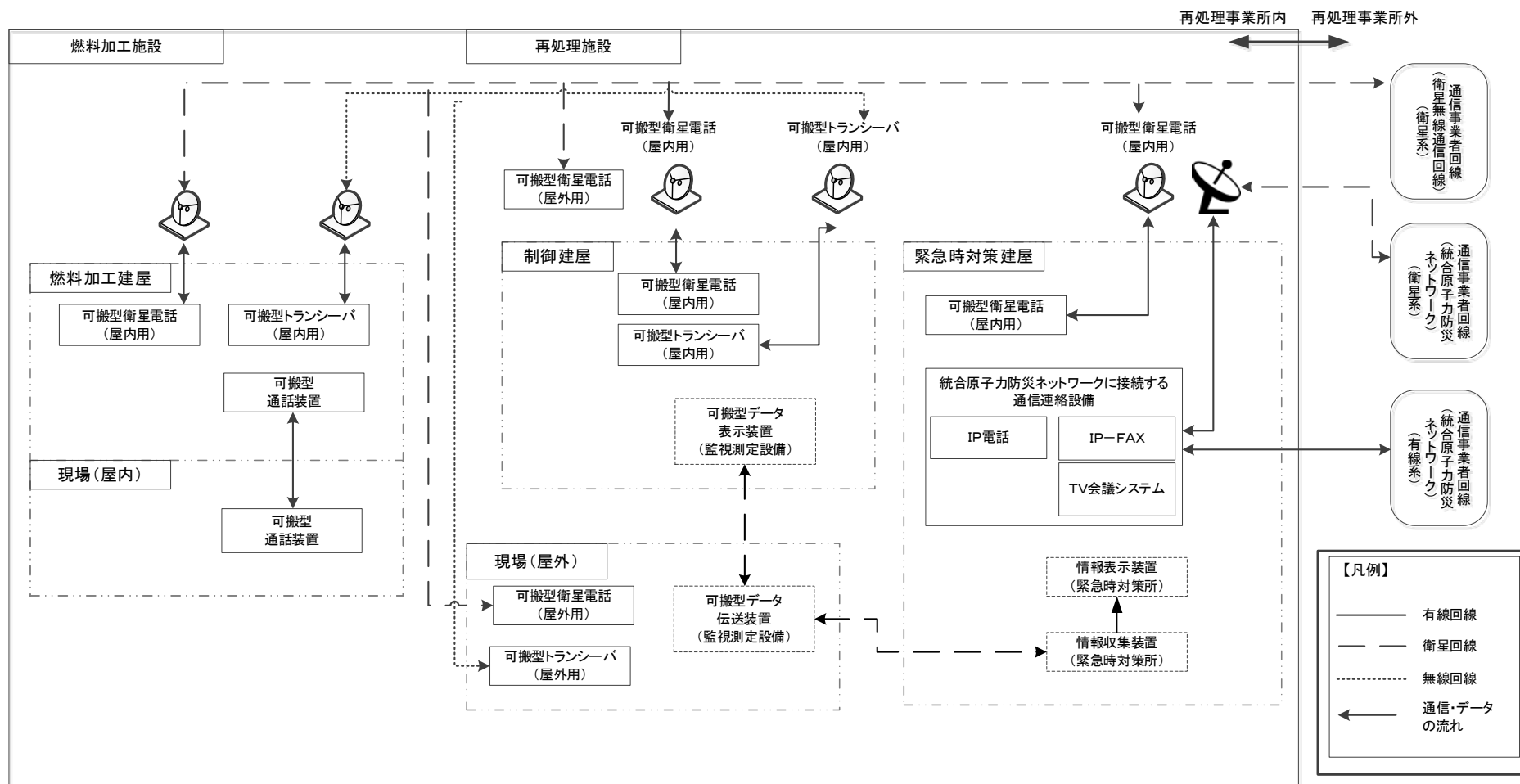
第 2. 1. 5 - 2 図 代替通信連絡設備の系統概要図
