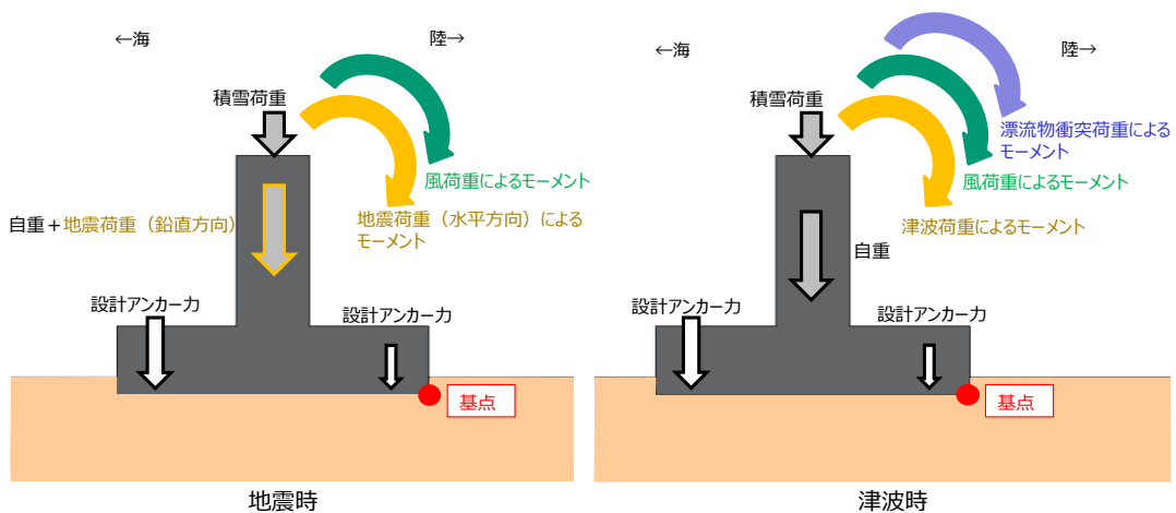
第 10-4-6 図 転倒の照査における荷重イメージ
