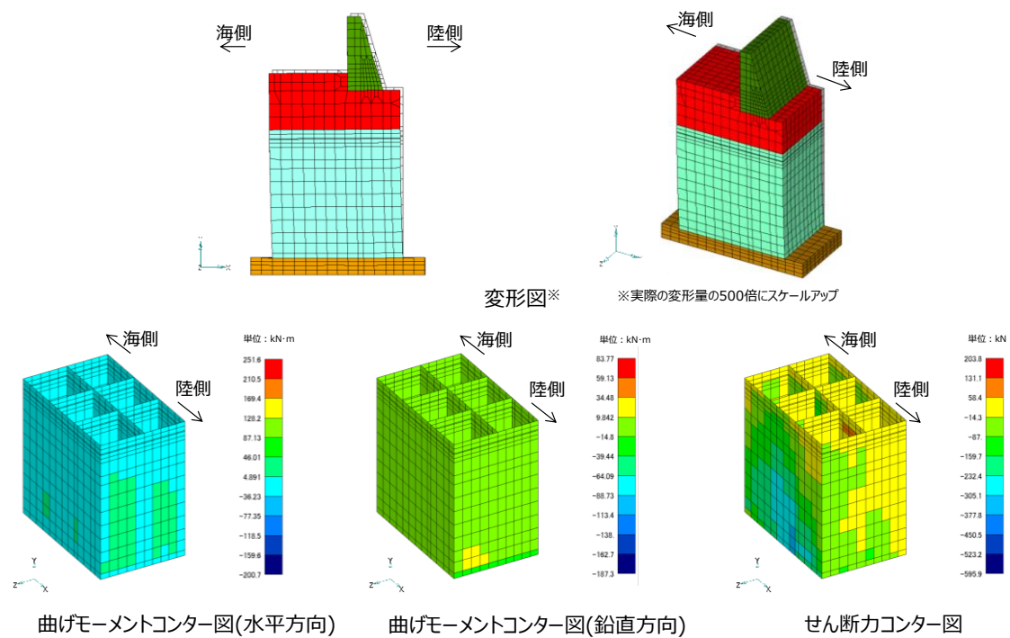
第10-5-11図 3次元静的FEM解析結果（輪谷部）
