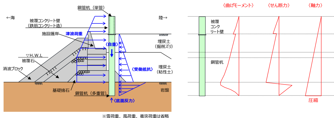
荷重図
