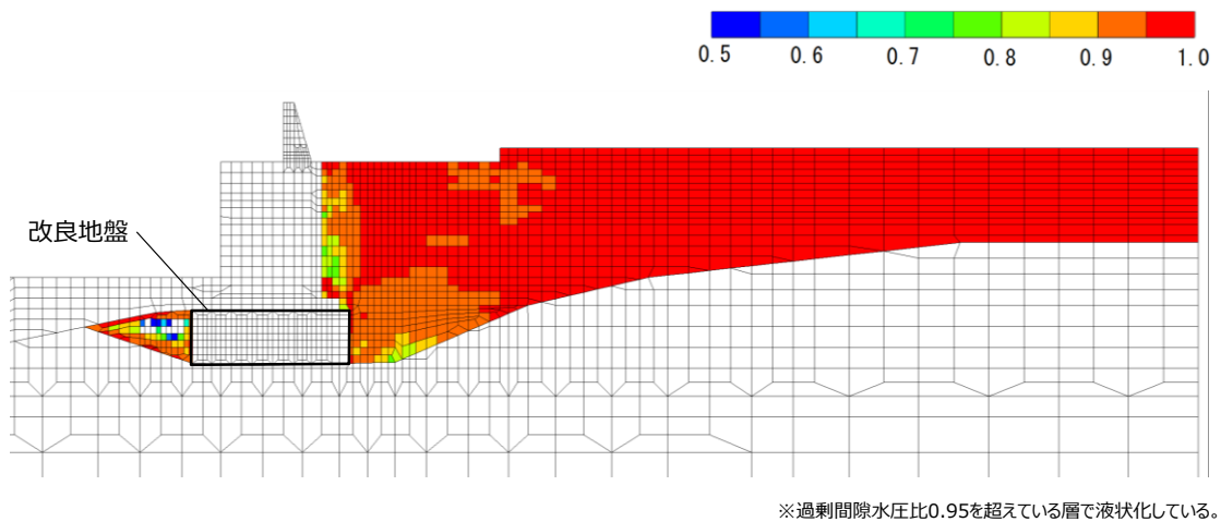
第 10-5-10 図 全時刻での過剰間隙水圧比分布
