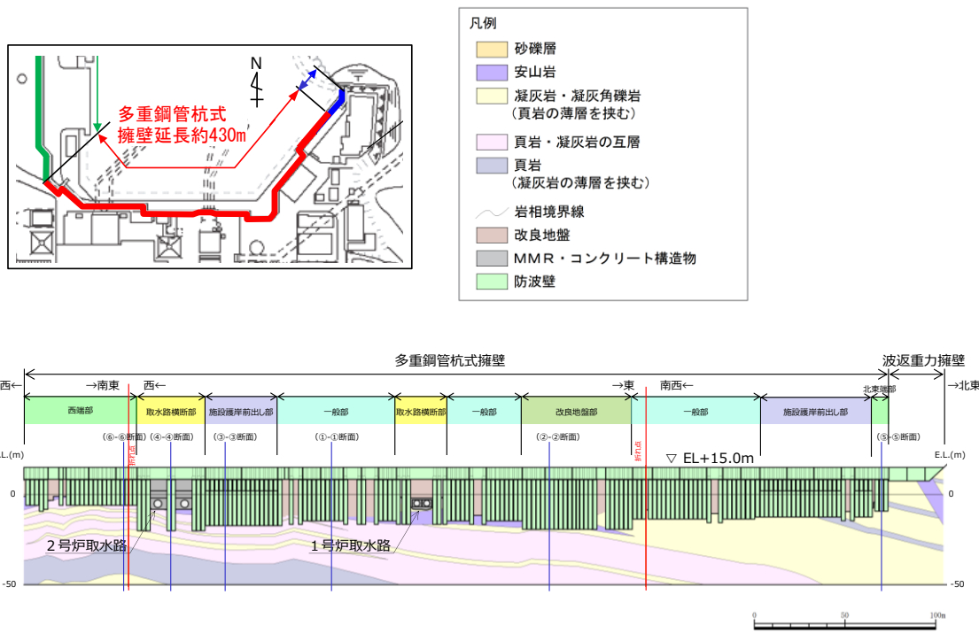
第 5-10 図 防波壁（多重鋼管杭式擁壁）の地質縦断図
