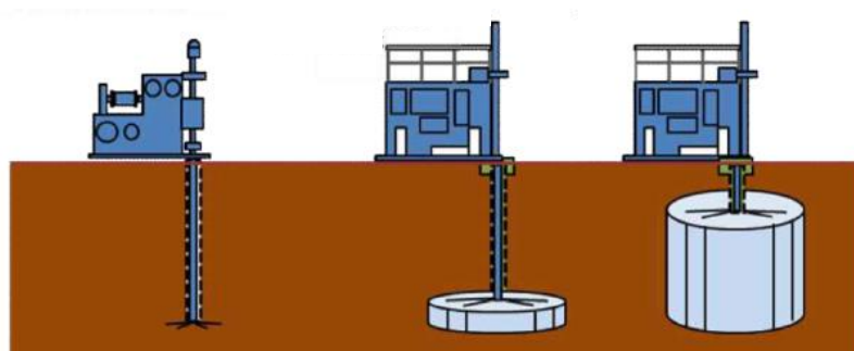
高圧噴射攪拌工法の施工イメージ
