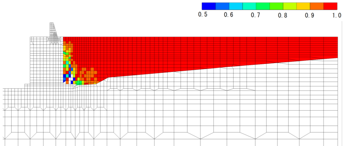
第 10-5-12 図 全時刻での過剰間隙水圧比分布
