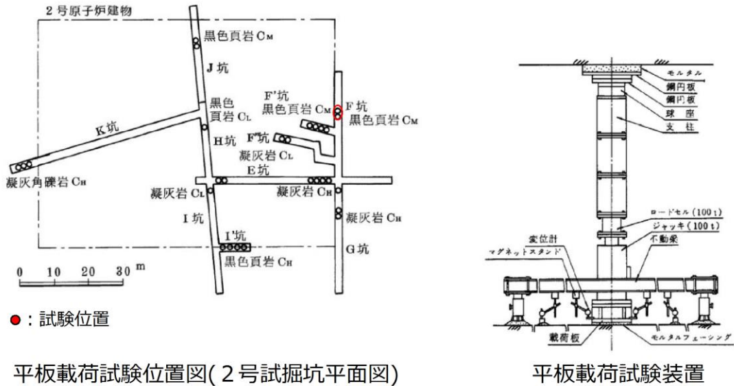
第 6-31 図 防波壁（鋼管杭式逆 T 擁壁）平板載荷試験概要
