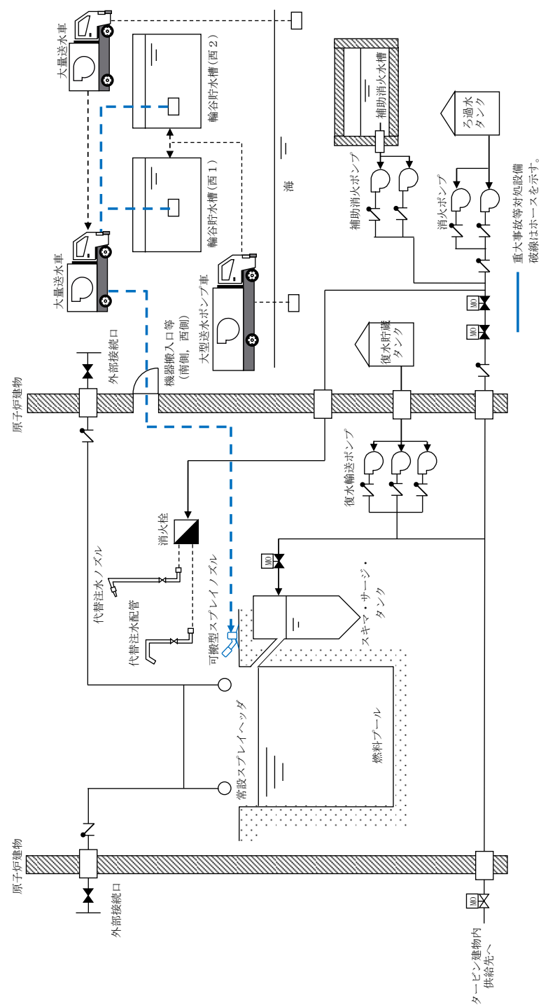
図1 燃料プールスプレイ系 (可搬型スプレイノズル) 燃料プールへ注水及びスプレイする場合の系統概要図
