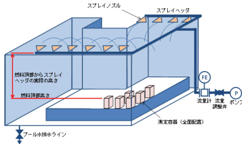
図6 試験設備概要図
